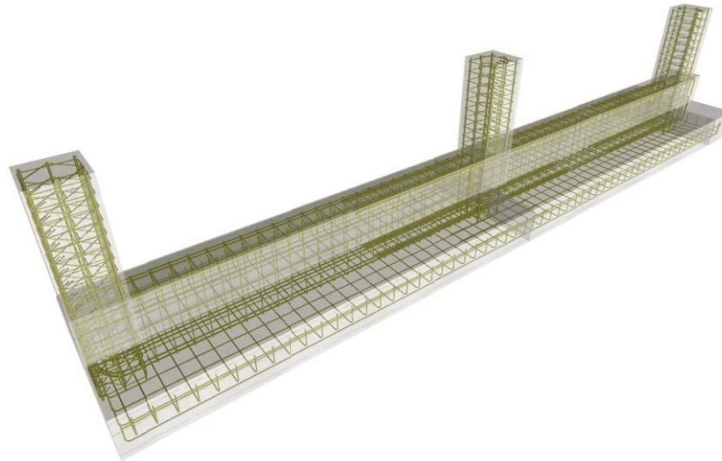
شکل ۱-۱۲ فونداسیون نواری
