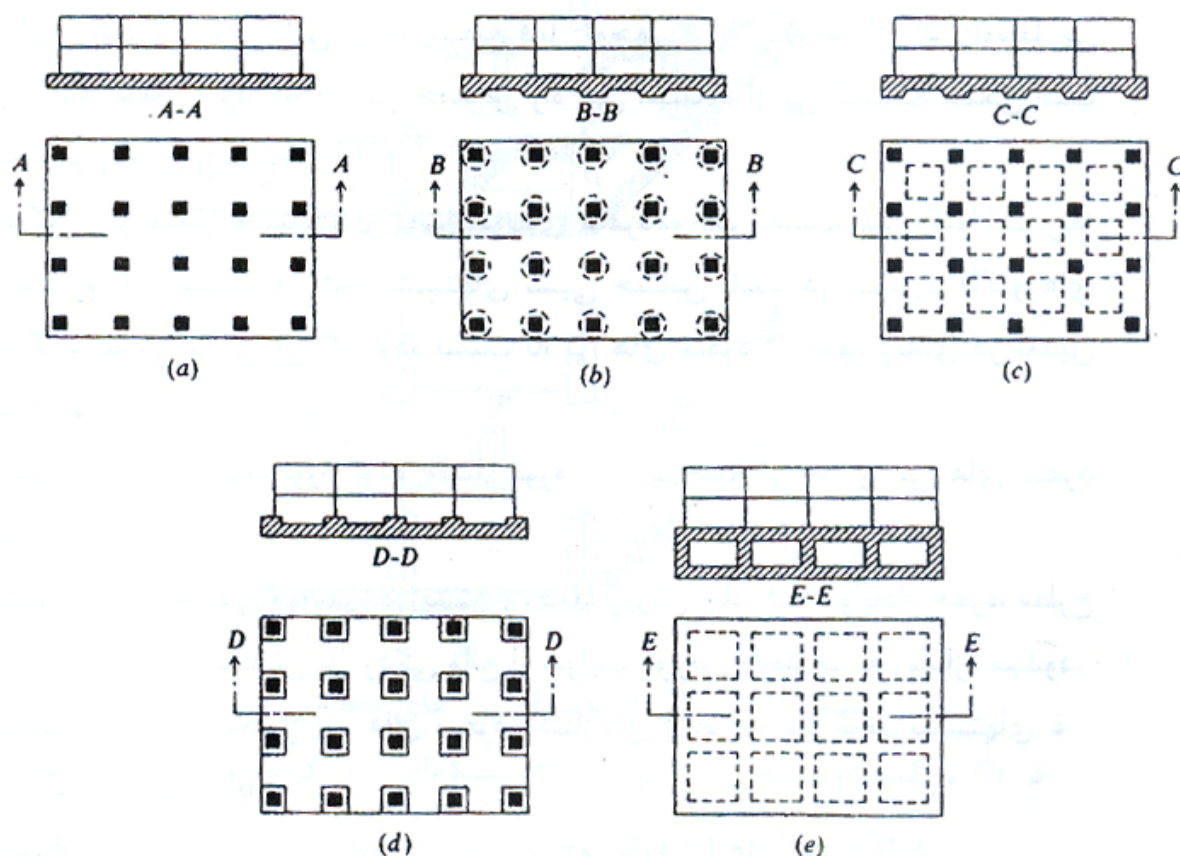
شکل ۱-۱۵ انواع مختلف فونداسیون های گسترده (a) سیستم دال تخت (b) سیستم قارچی (در بالا یا پایین) (c) سیستم دال دیوار (d) سیستم جعبه ای (e) دال کف، دال سقف و دیوارهای میانی و جانبی
