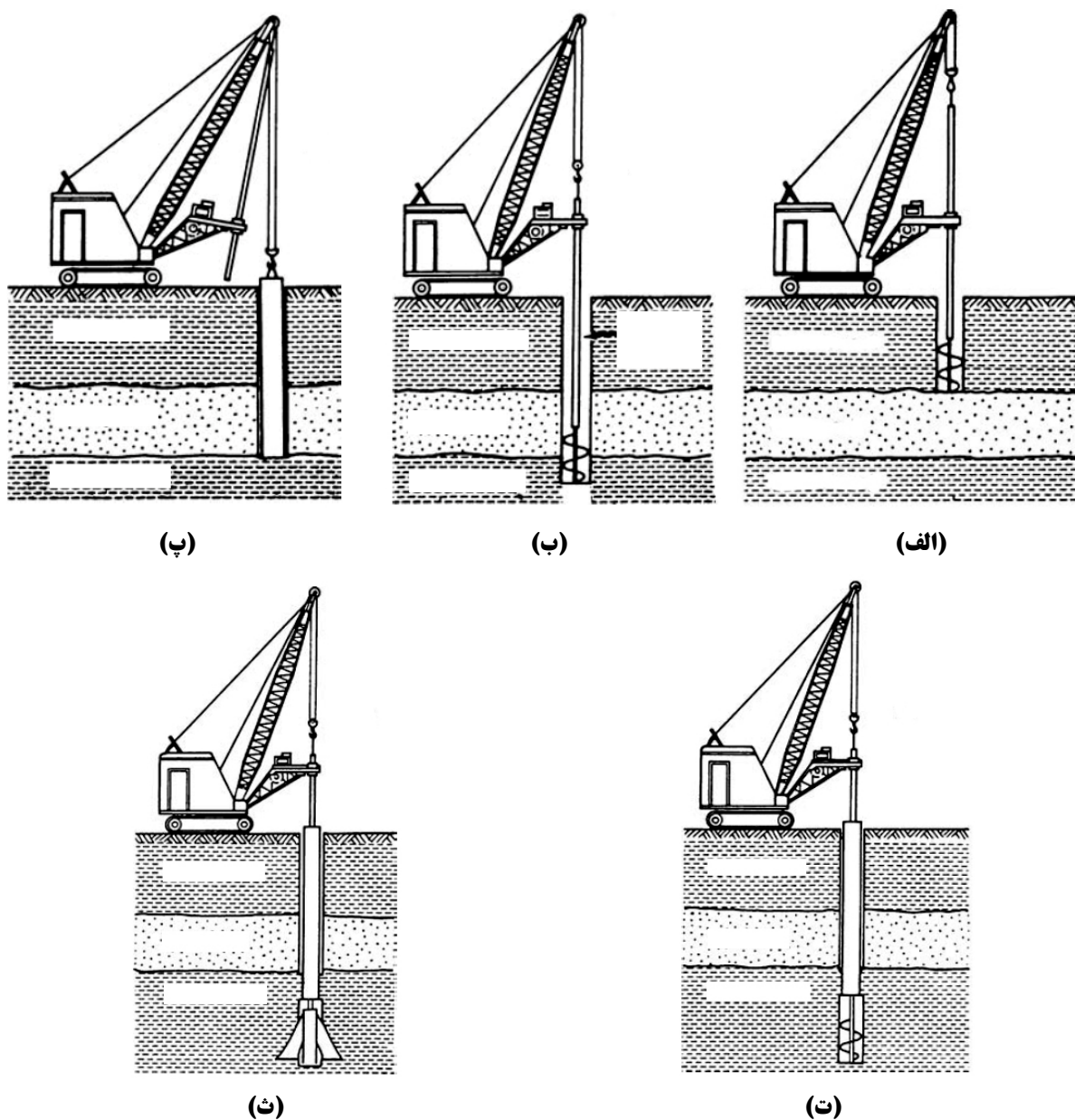
شکل ۱-۱۹ روش اجرای پایه های عمیق
