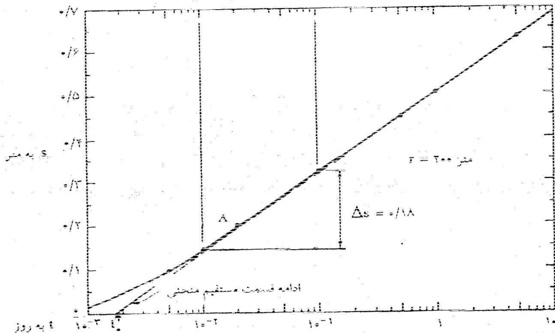
شکل (۱۸-۴) تغییرات S بر حسب \log t برای داده‌های جدول (۲-۴) و r = 200 متر برای
