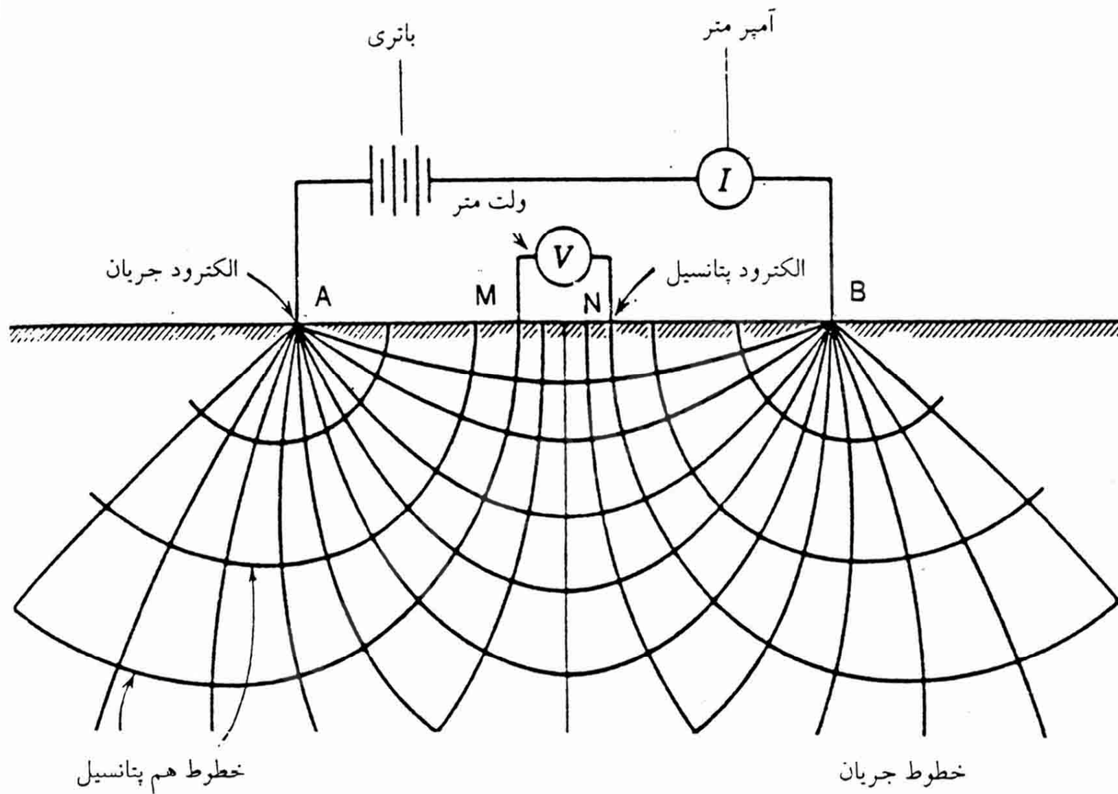
شکل ۱۰-۳ - الکتروودهای جریان و پتانسیل برای اندازه گیری مقاومت ویژه ظاهری
