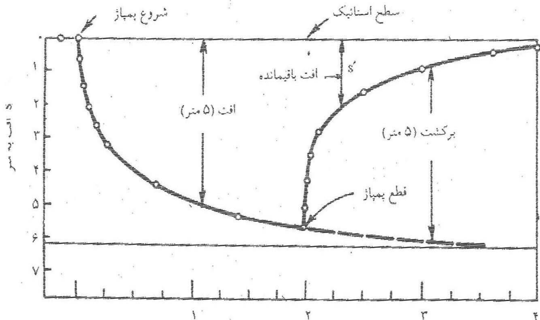
شکل ۴-۱۹- منحنی افت و برگشت در یک چاه که به مدت ۴۸ ساعت با دبی ثابت پمپاژ
