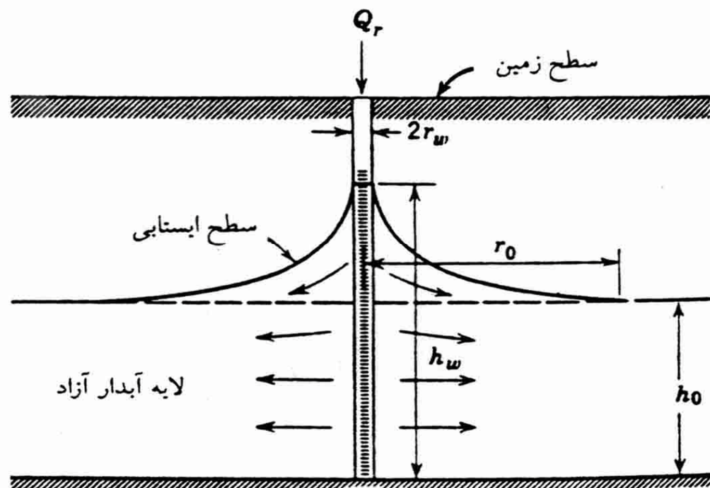
شکل ۵-۷ جریان شعاعی در اطراف چاههای تغذیه: الف: در لایه آبدار تحت فشار، ب - در لایه آبدار آزاد
