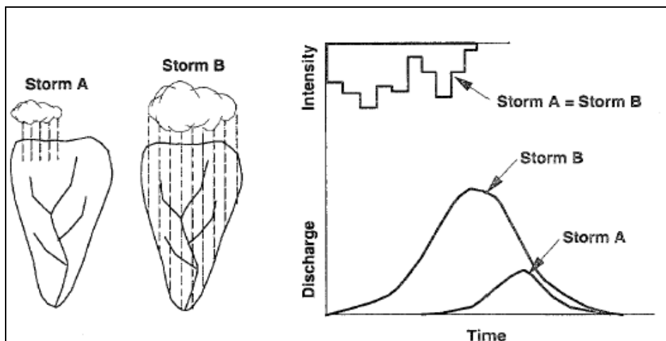
شکل 2-4 تاثیر وسعت محدوده بارندگی در یک حوضه آبریز برای دو رگبار مختلف
