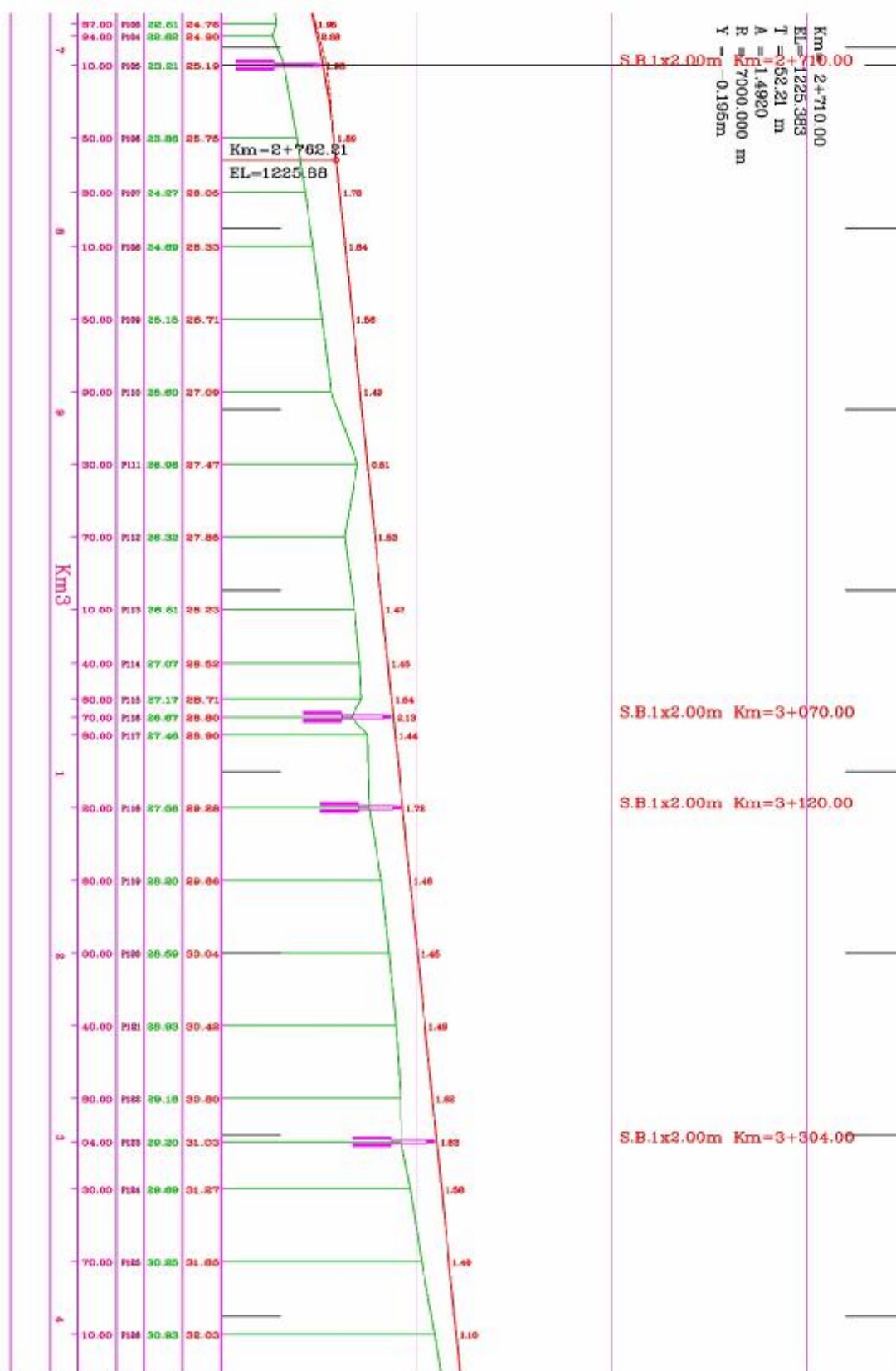
شکل 1-3- پروفیل طولی مسیر و جانمایی آبروها در یک منطقه دشت [مرجع شماره 10]
