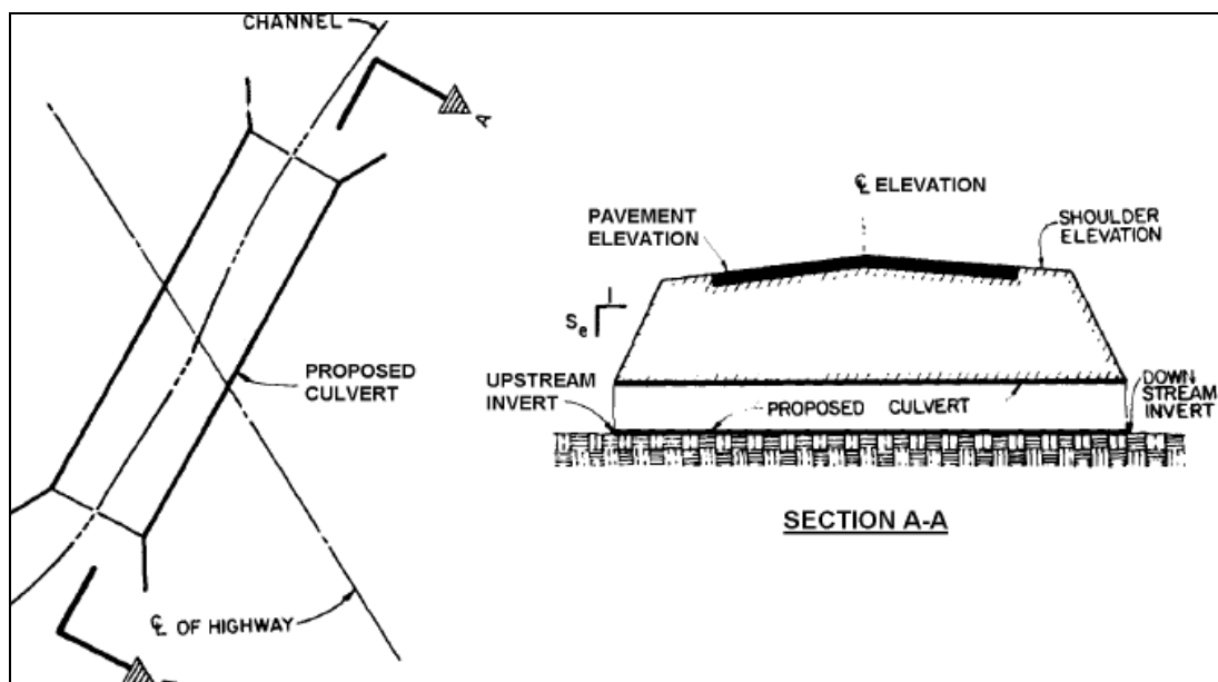
شکل 7-4 تیپ مقطع عرضی مسیر و طول آبرو
