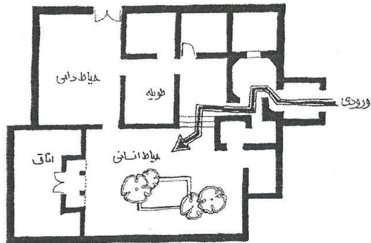
پلان با هشتی با انواع شکست های ورودی
