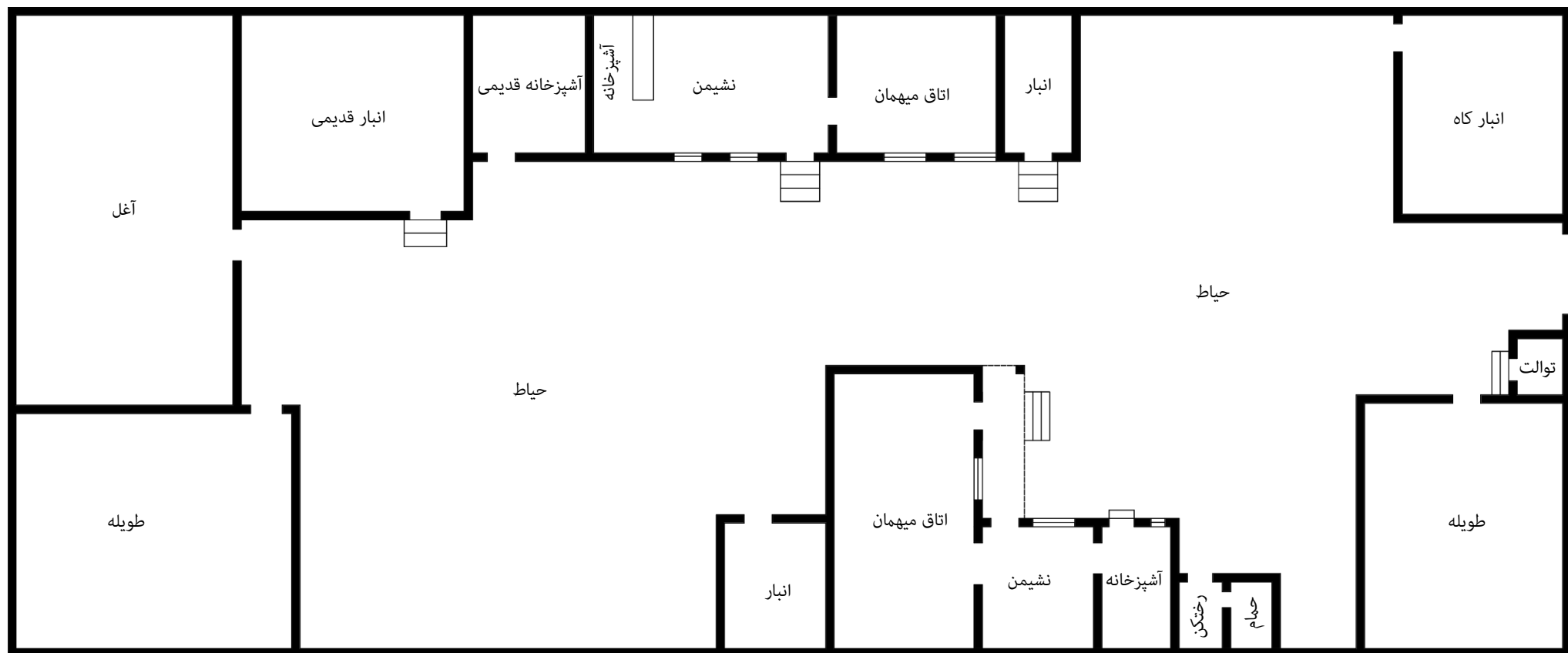
پلان - مقیاس ۱/۲۰۰
