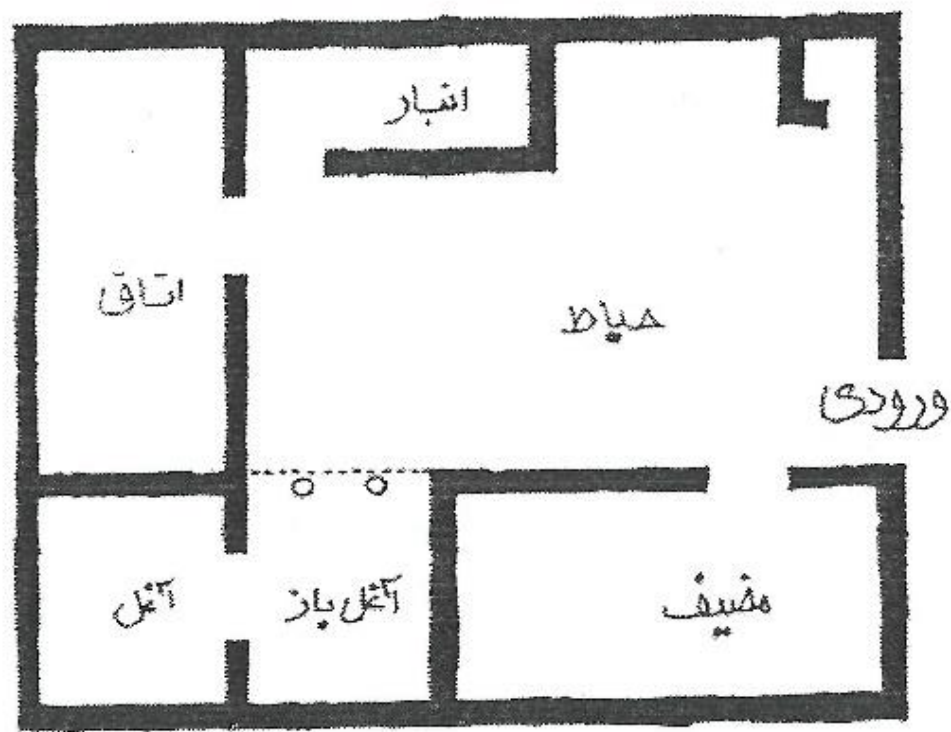
پلان یک خانه در ناحیه دشت آزادگان و محل مضیف آن
