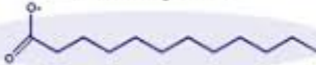
Free fatty acid
