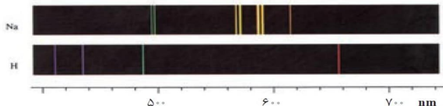
شکل ۵ طیف نشری خطی عنصرهای سدیم و هیدروژن
