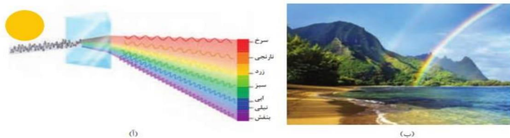
شکل ۱۴-۱) نور خورشید هنگام عبور از منشور تجزیه می شود. ب) رنگین کمان، گستره‌ای از رنگ‌های سفید تا بنفش را در برمی گیرد.
