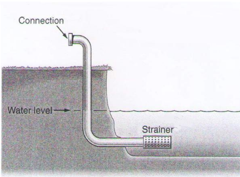
شکل شماره 1-2: لوله‌های آبیگیری ثابت
