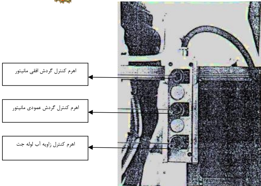
شکل شماره 2-25: تابلوی اهرم‌های کنترل از راه دور مانیتور در بالابر "برونتو"
