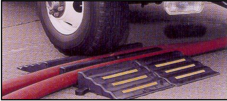
شکل شماره 2-14: پل محافظ لوله
