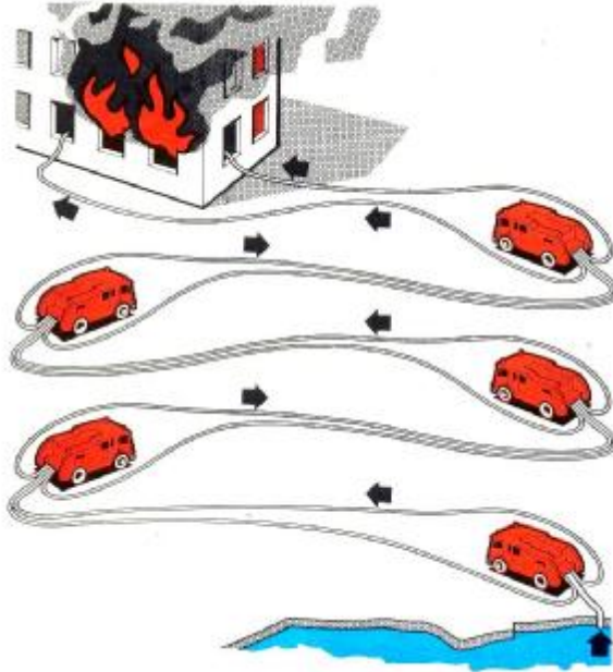
شکل شماره 5-1: طرح نمایش روش رله مدار بسته
