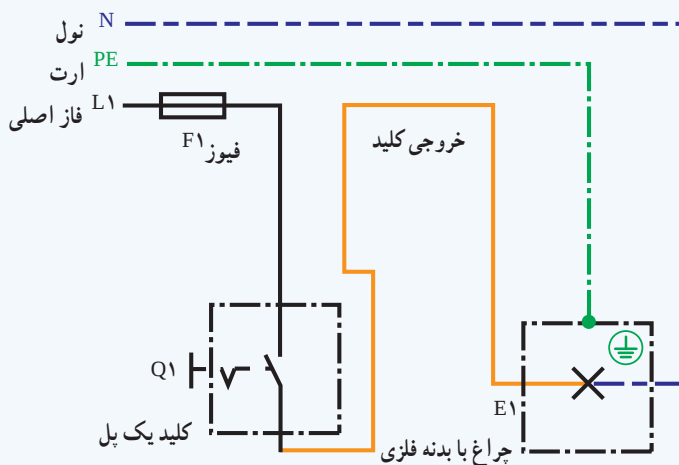
شکل ۲۰-۲ نقشه شمای حقیقی مدار کلید یک پل
