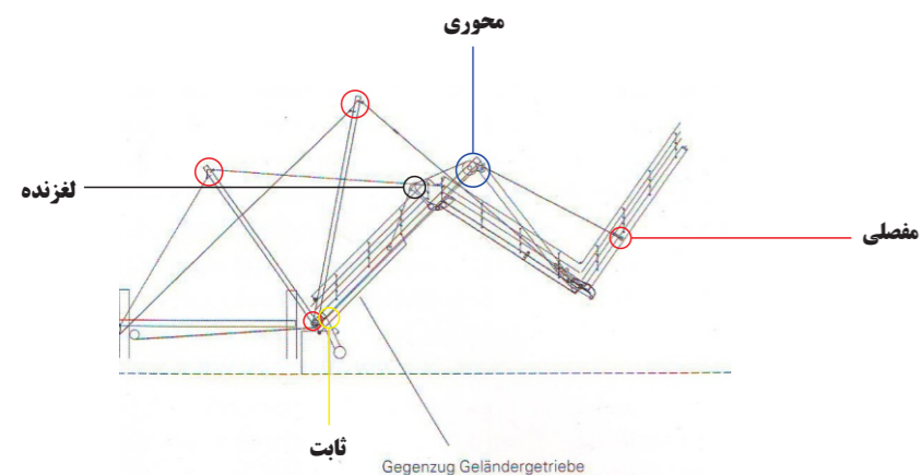
نمای باز پل
