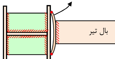
شکل (32): پیوستگی نامناسب تیر به ستون در صورت استفاده از ورق تقویتی روی ستون
