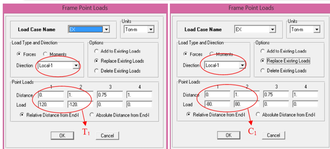
شکل (24): اختصاص نیروهای T_1 و C_1 به مهاربندها
