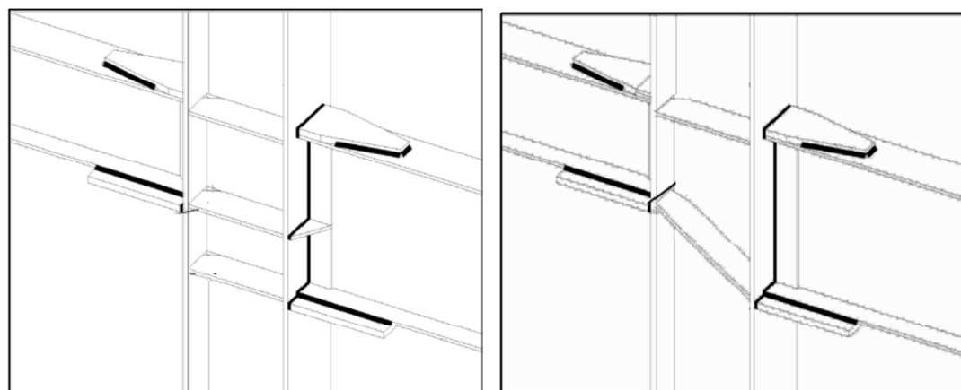
شکل (33): دتایل اجرایی ورق پیوستگی ستون برای تیرهای با ارتفاع متفاوت
