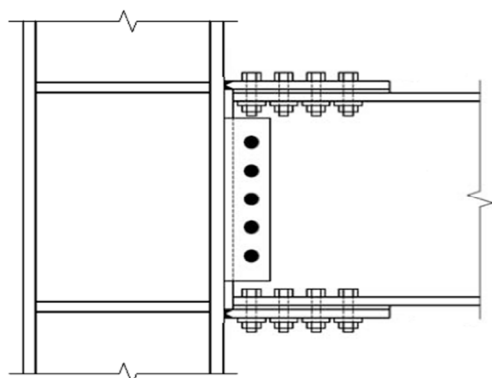
اتصال با ورق روسری و زیرسری پیچی
