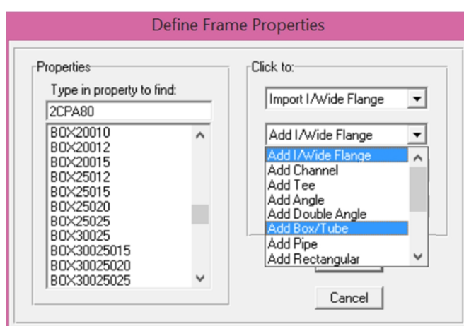
شکل (31): معرفی مقاطع H و Box در نرم افزار
