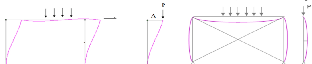
شکل (1): آثار مرتبه دوم P-\delta و P-\Delta
