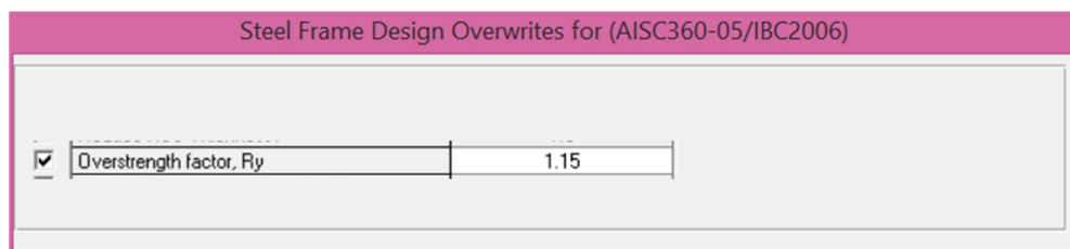
شکل (42): اختصاص ضریب تولیدات فولاد ( R_y ) اعضاء
