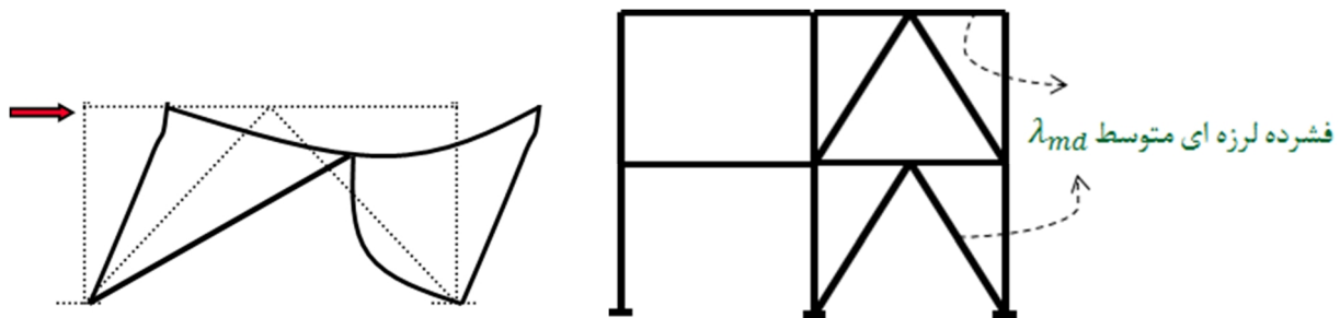
شکل (11): مقطع مناسب دهانه مهاربند 7 و 8 شکل (12): تغییر شکل های فرا ارتجایی مهاربند 7 و 8
