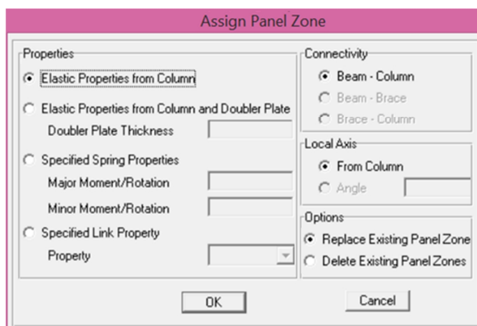
شکل (37): در نظر گرفتن اثر تغییر شکل برشی چشمه اتصال در نرم افزار
