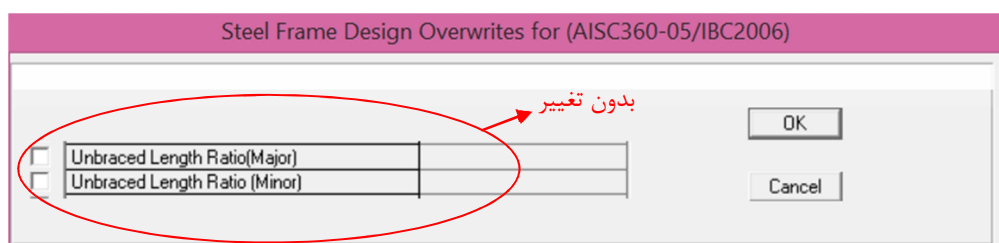
شکل (35): استفاده از پیش فرض نرم افزار برای مهار بال جانبی تیرهای عرشه فولادی
