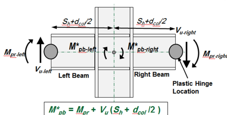
شکل (40): تصاویر لنگرهای خمشی تیرها در گره اتصال
