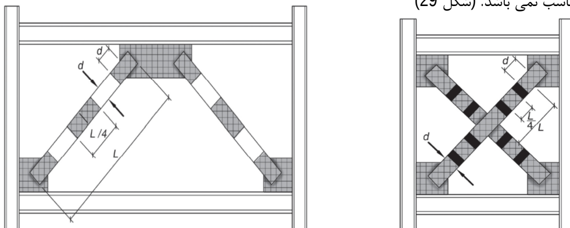
شکل (29): نواحی محافظت شده مهاربند های X و 7 و 8
