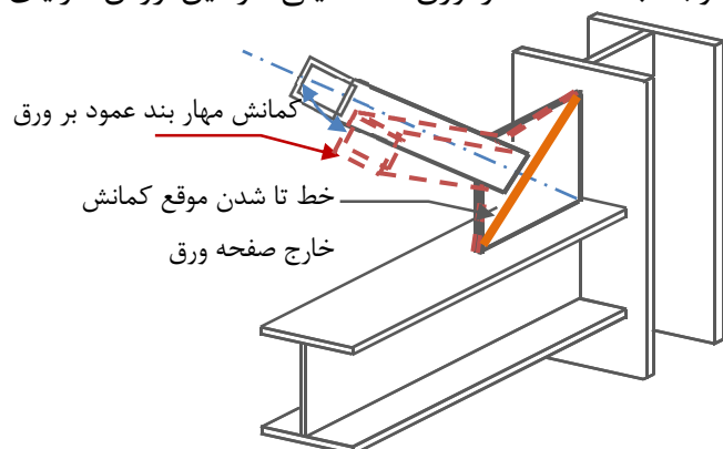
شکل (26): فاصله خطی 2t و بیضوی 8t برای آزادی دورانی غیر الاستیک اتصال مهاربندی ویژه
