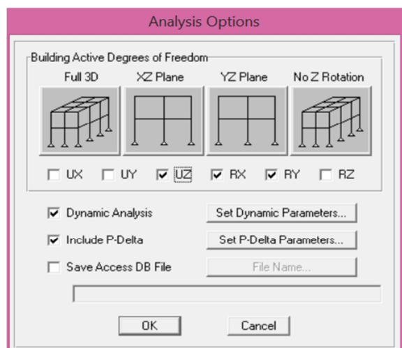
شکل (25): حذف درجات آزادی
