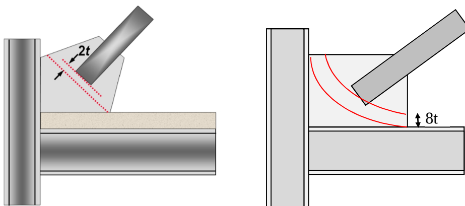
شکل (27): فاصله خطی 2t و بیضوی 8t برای آزادی دورانی غیر الاستیک اتصال مهاربندی ویژه
