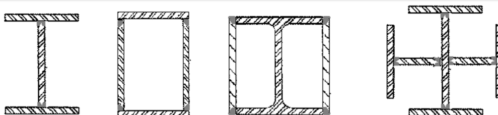
شکل (30): مقاطع مناسب برای ستون ها در سیستم قاب های خمشی
