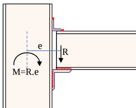
شکل (3): لنگر جزئی ستون ناشی از خروج از مرکزیت عکس العمل تیر نسبت به محور ستون
