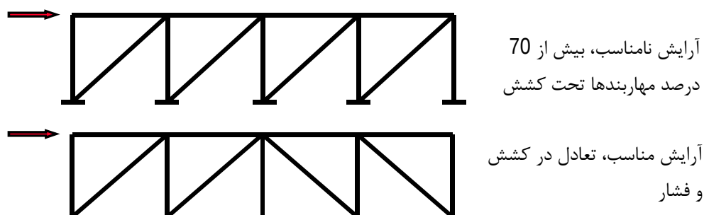
شکل (21): آرایش مناسب مهاربندها در یک محور
