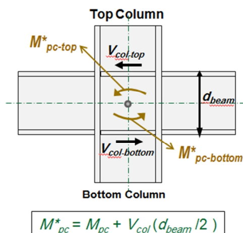
شکل (41): لنگرهای خمشی ستون‌ها بالا و پایین گره اتصال
