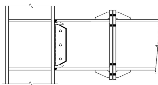
اتصال مستقیم جوشی با وصله فلنجی
