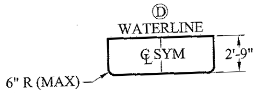
SECTION d-d
