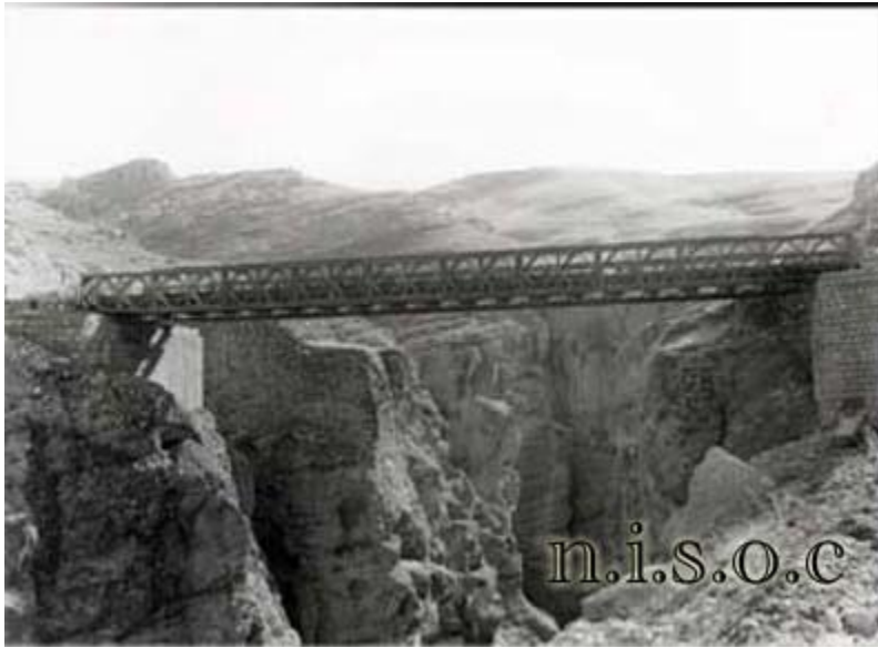
پل فلزي عبور خط لوله
