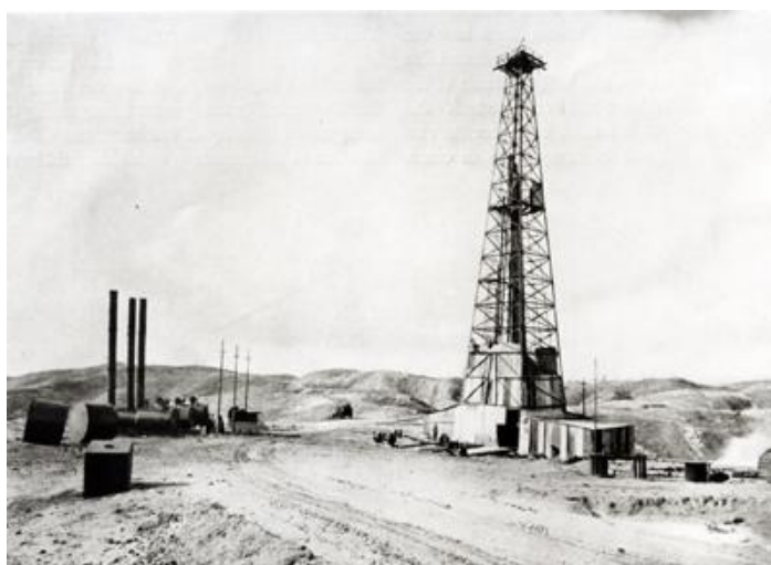
اولین دکل حفاری در مسجد سلیمان
