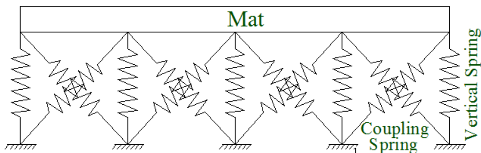
شکل ۲۲- مدل سازی فنرهای کوپله
