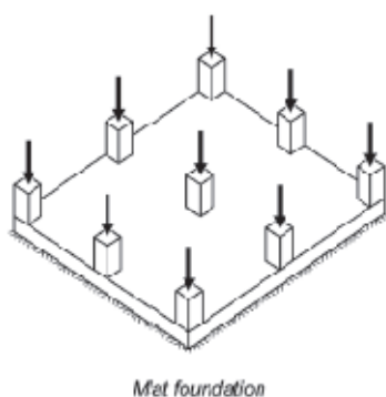
شکل ۷- پی گسترده
