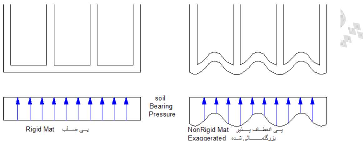
شکل-۱۸-مقایسه توزیع تنش در زیر پی صلب و غیر صلب
