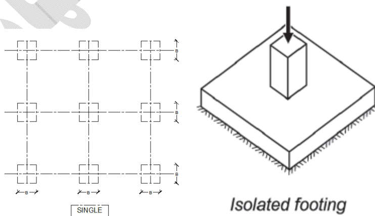
شکل ۳- پی تکی
