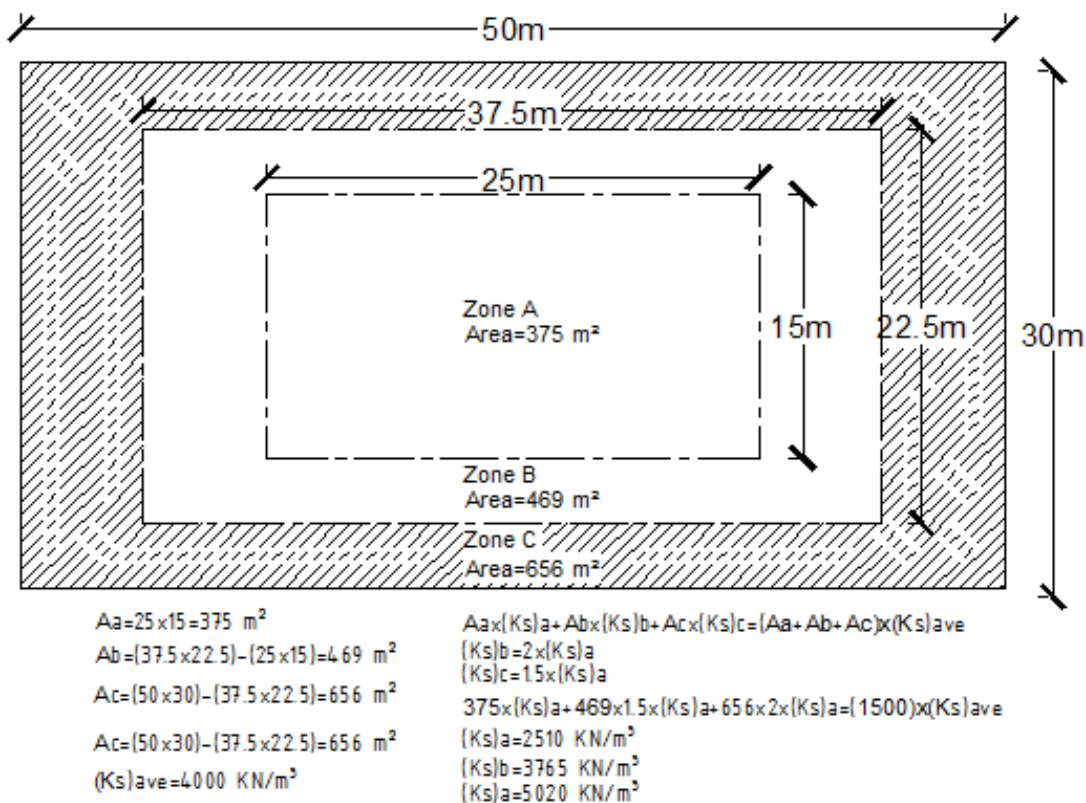
شکل ۲۶- پی گسترده در روش شبه کوپل-مثال عددی
