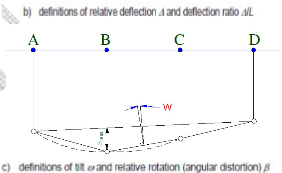
شکل ۳۳- مفهوم نشست های تفاضلی و چرخش
