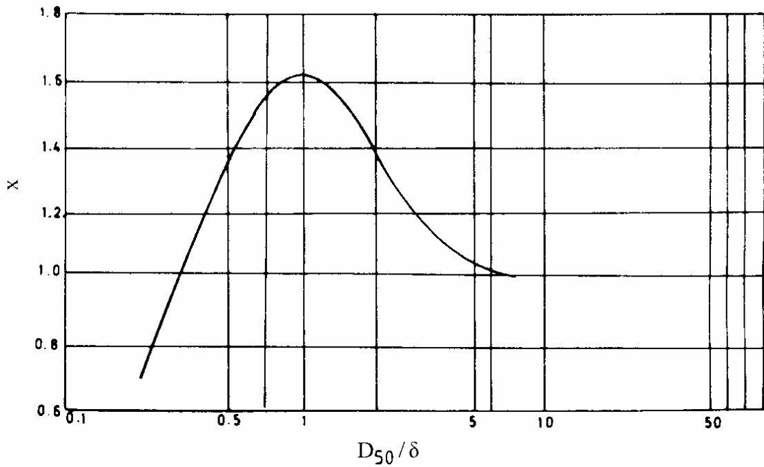
شکل ۲-۷- نمودار تغییرات پارامتر X بر حسب پارامتر \frac{D_{50}}{\delta}
