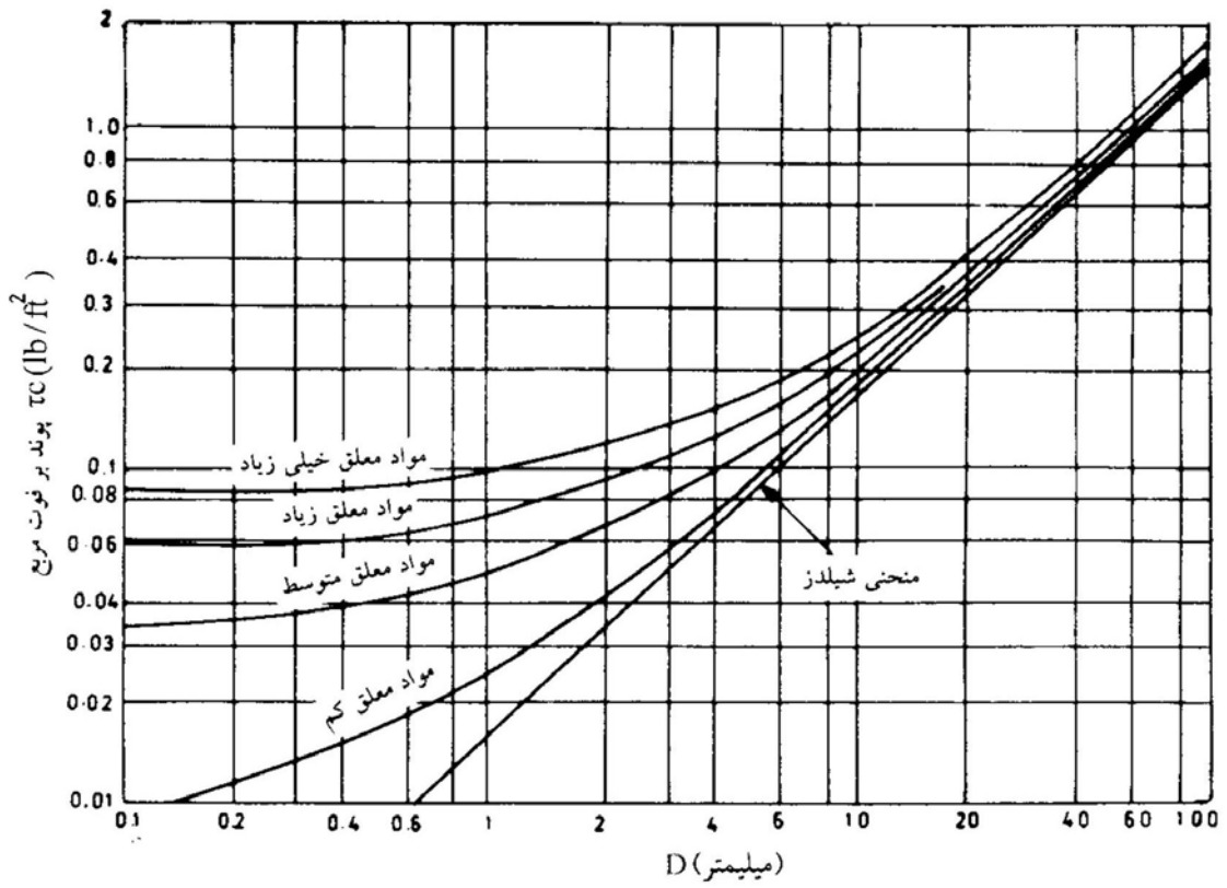
شکل ۱-۷- نمودار تغییرات تنش برشی بحرانی ( \tau_c ) بر حسب قطر مواد بستر D_{50}
