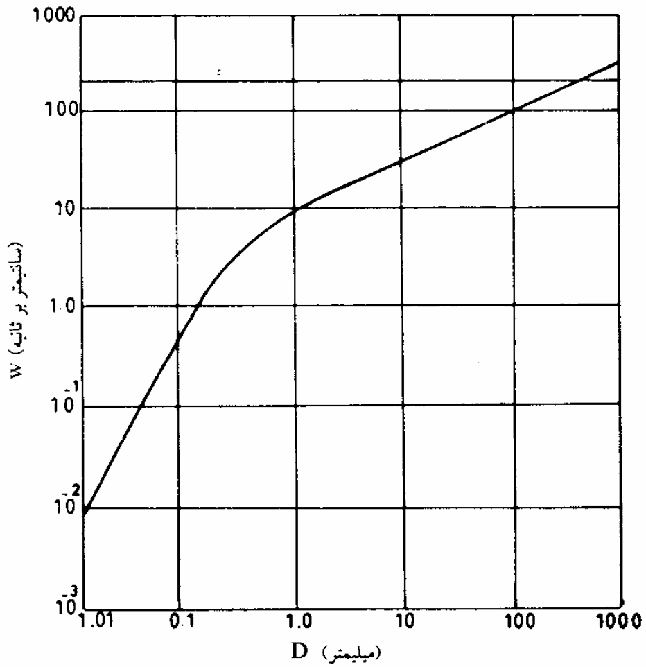
شکل ۵-۷- نمودار تغییرات سرعت سقوط دانه‌ها ( w ) بر حسب قطر دانه ( D )
