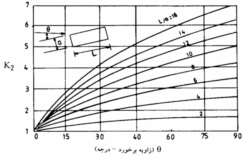
شکل ۴-۷- ضریب تصحیح K_2 بر حسب \theta برای پل‌های مستطیلی
