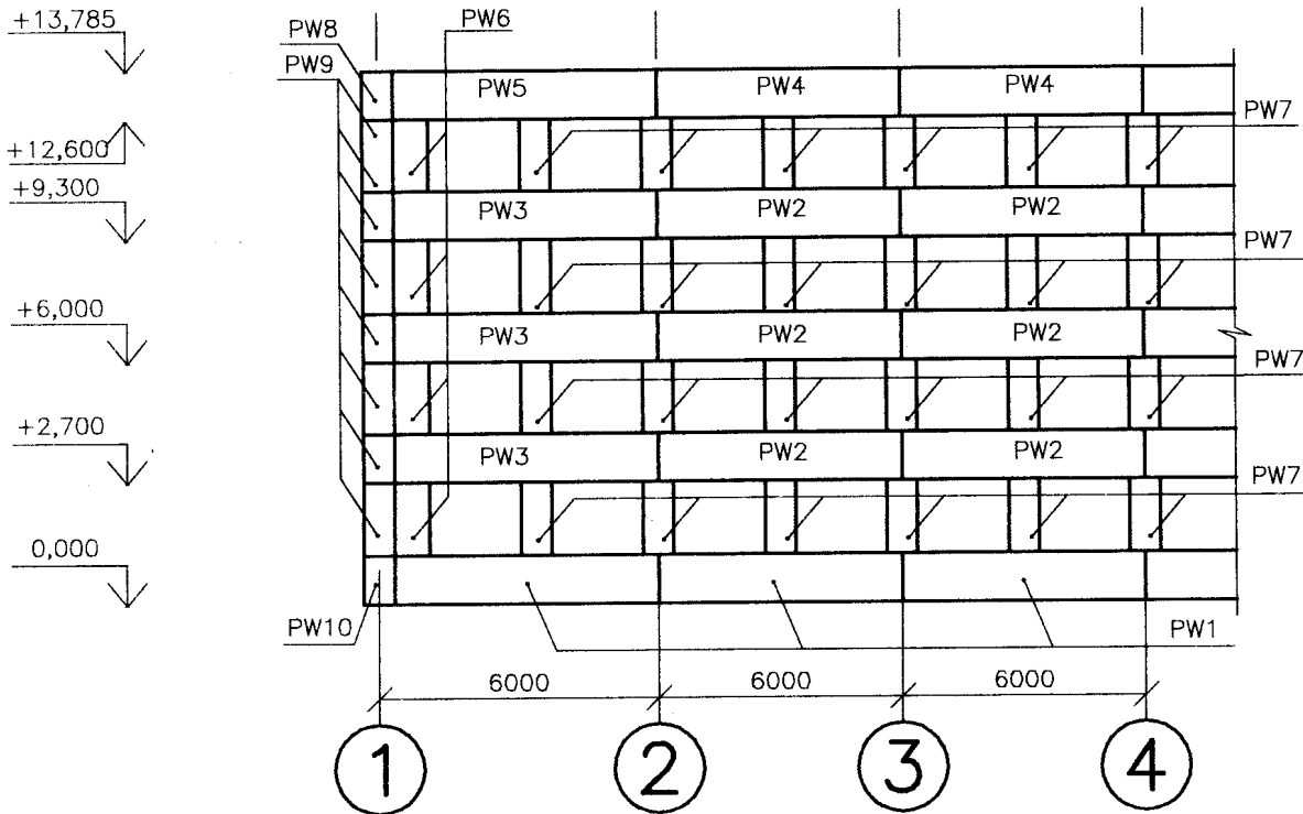
شکل ۵- مثالی برای نقشه جانمایی دیوارهای پیش‌ساخته. (نما)
