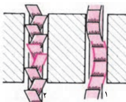
۱- چپ و راست نمودن دندانه ها ۲- موج دادن به لبه تیغه اره
