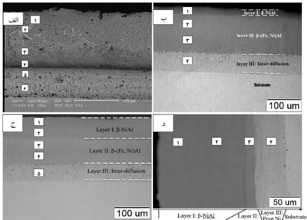
شکل ۳. الف) تصویر میکروسکوپ الکترونی روبشی فولاد زنگ نزن آلومینایز شده در دمای 1080^{\circ}\text{C} به مدت ۲/۵ ساعت و در پودر با ترکیب 88\% \text{Al}_2\text{O}_3 + 10\% \text{Al} + 2\% \text{NH}_4\text{Cl} (ب، ج و د) به ترتیب پوشش آلومینایز تشکیل شده بر روی نمونه‌های با ضخامت نیکل اولیه ۱۰، ۲۰ و ۵۰ میکرون.
