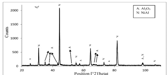
شکل ۵-الف) رابطه‌ی تغییر وزن با زمان در نمونه‌ی T1080 در بازه‌ی ۲۴ تا ۱۵۷ ساعت. ب) نتایج XRD نمونه‌ی T1080 بعد از اکسیداسیون.
