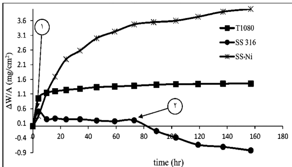
شکل ۴- منحنی تغییرات وزن نمونه‌های آلومینایز شده در دمای بالا، فولاد زنگ نزن و فولاد زنگ نزن آبرکاری شده.
