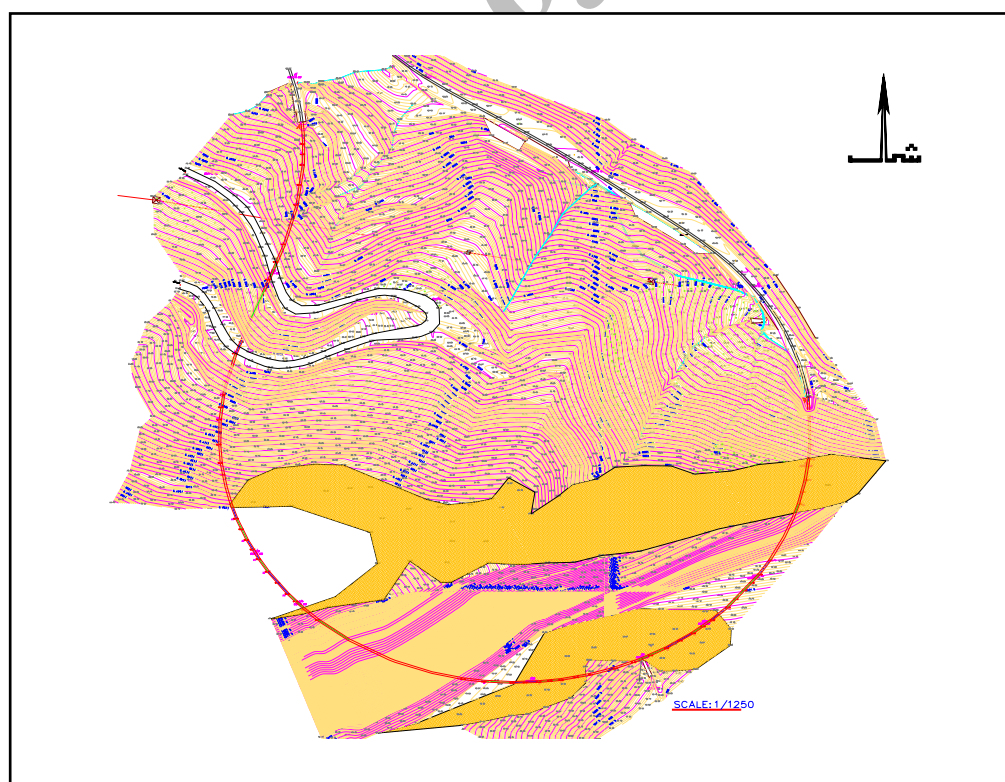
شکل ۳. پلان مسیر تونل ۱۰۲ راه آهن لرستان [۲]
