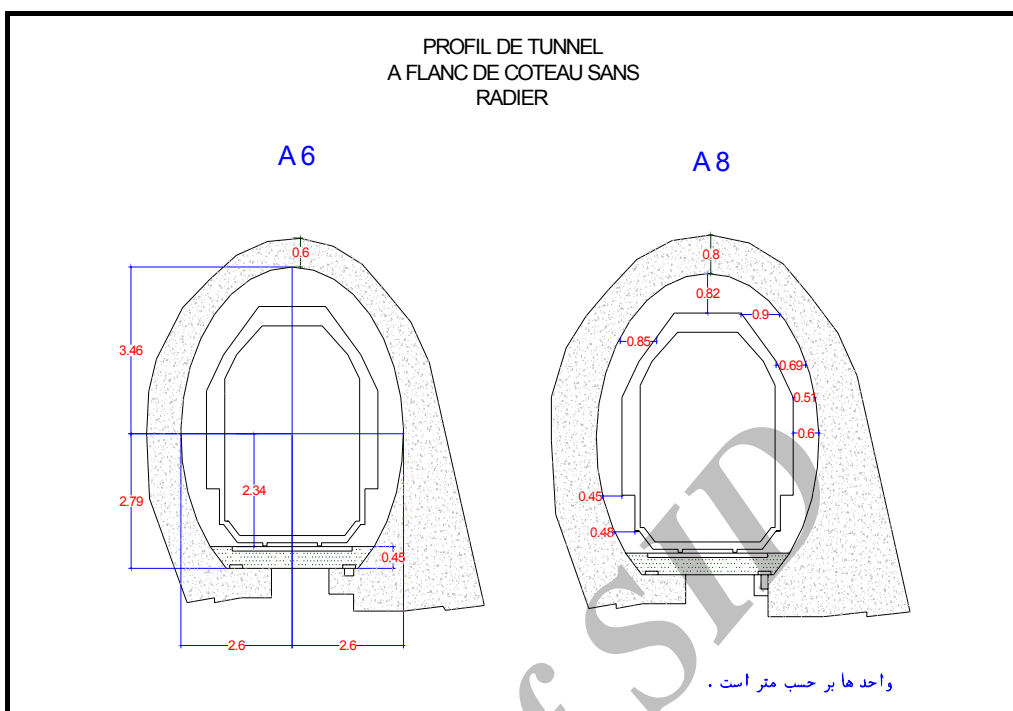
شکل ۲. مقطع عرضی تونل [۲]
