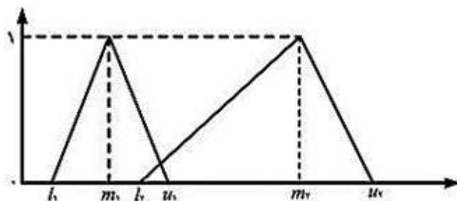
نمودار ۱. اعداد مثلثی M_2 و M_1
