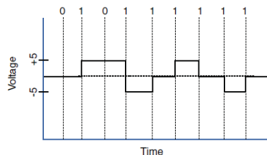
شکل ۴-۳ State Transition Modulation
