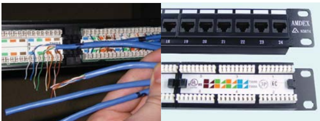
شکل ۲۳-۳: Patch Panel
