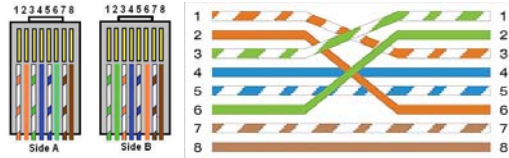
شکل ۵-۶: کابل Cross-Over
