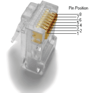
شکل ۳-۵ شماره پین‌های کانکتور RJ45
