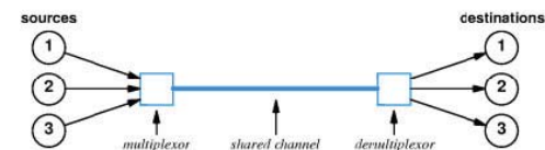
شکل ۴-۴ مالتی پلکسینگ
