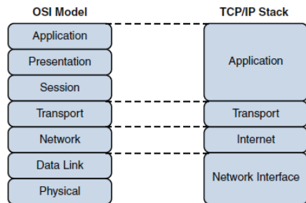
شکل ۴-۷: مقایسه OSI و TCP/IP
