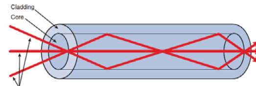
شکل ۳-۱۴: انتشار نور در فیبر چند حالت
