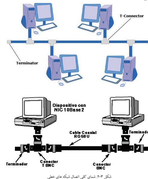
شکل ۲-۳: شمای کلی اتصال شبکه های خطی
