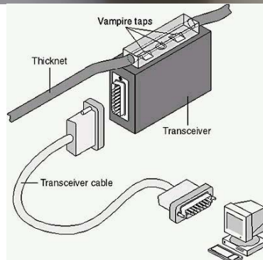
شکل ۱-۵: کانکتور Vampire Tap
