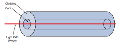
شکل ۳-۱۵: انتشار نور در فیبر تک حالت
