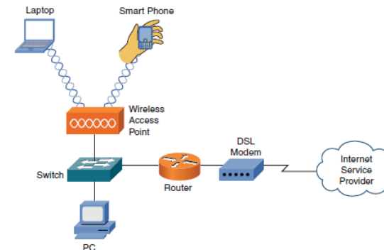
شکل ۴-۸: Wireless Access Point
