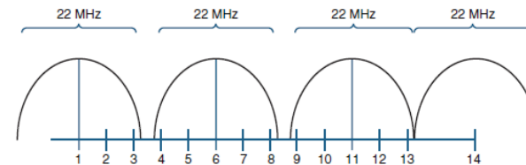
شکل ۸-۷: باند فرکانسی 2.4GHz
