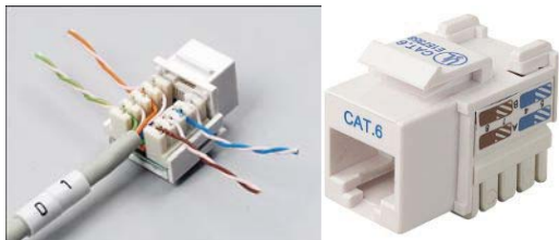
شکل ۳-۲۸: Keystone
