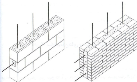
دیوار بلوک سیمانی مسلح
