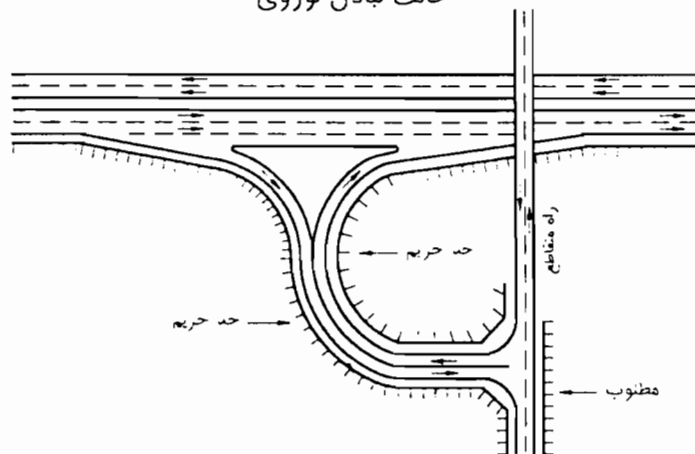
محدوده کنترل دسترسی در حالت مالکیت خصوصی در داخل گردراه
