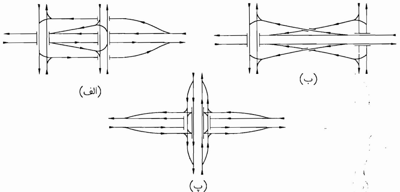
شکل ۷-۸ تبادلی لوزوی با تسهیلات (سازه‌های) اضافی
