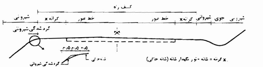
شکل ۶-۲ اجزاء نیمرخ عرضی راه چهار خطه مجزا و راه دو خطه دو طرفه
