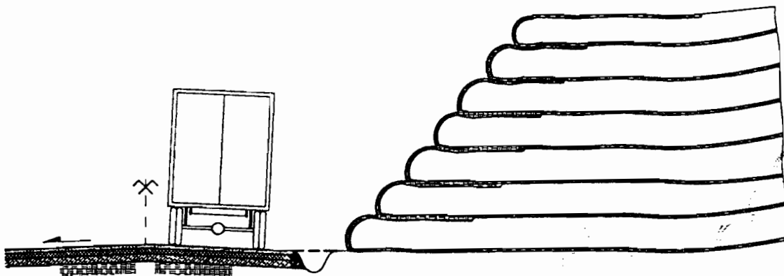
شکل ۲۹-۵ خاک مسلح
