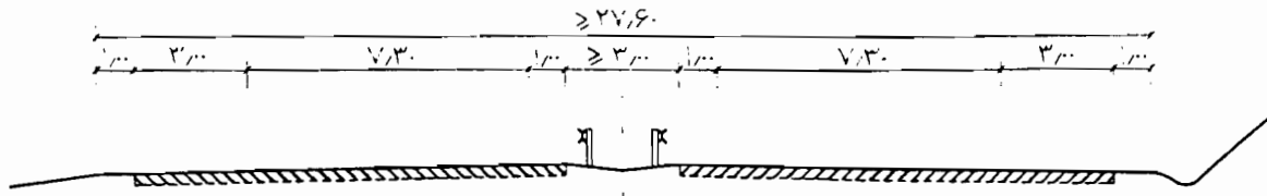
چهار خطه با جزیره وسط بدون روبه
