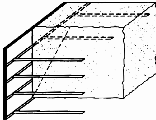
شکل ۲۹-۵ خاک مسلح
