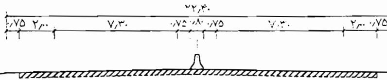
شش خطه با جزیره وسط بدون روبه
