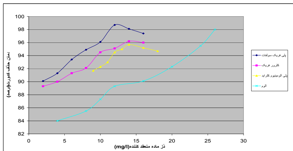
شکل 3- الف-مقایسه عملکرد چهار ماده منعقد کننده در حذف کدورت 320NTU
