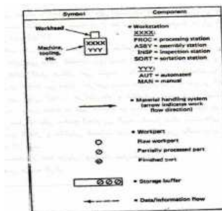
شکل ۵-۱. علائمی که در نمودار های سیستم های تولید به کار می روند.
