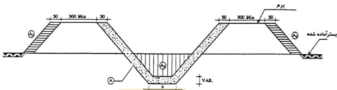
شکل ۵-۶. شمالی مقطع خاکبرداری
