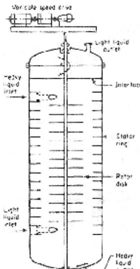
شکل 2-36- استخراج کننده با دیسک چرخان RDC
