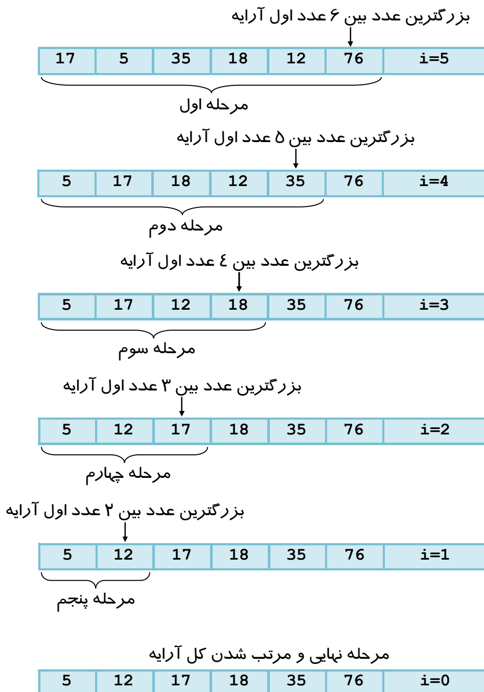
شکل ۷-۴: نحوه‌ی رسیدن بزرگ‌ترین عدد به انتهای آرایه‌ی به طول i+1 در هر مرحله
