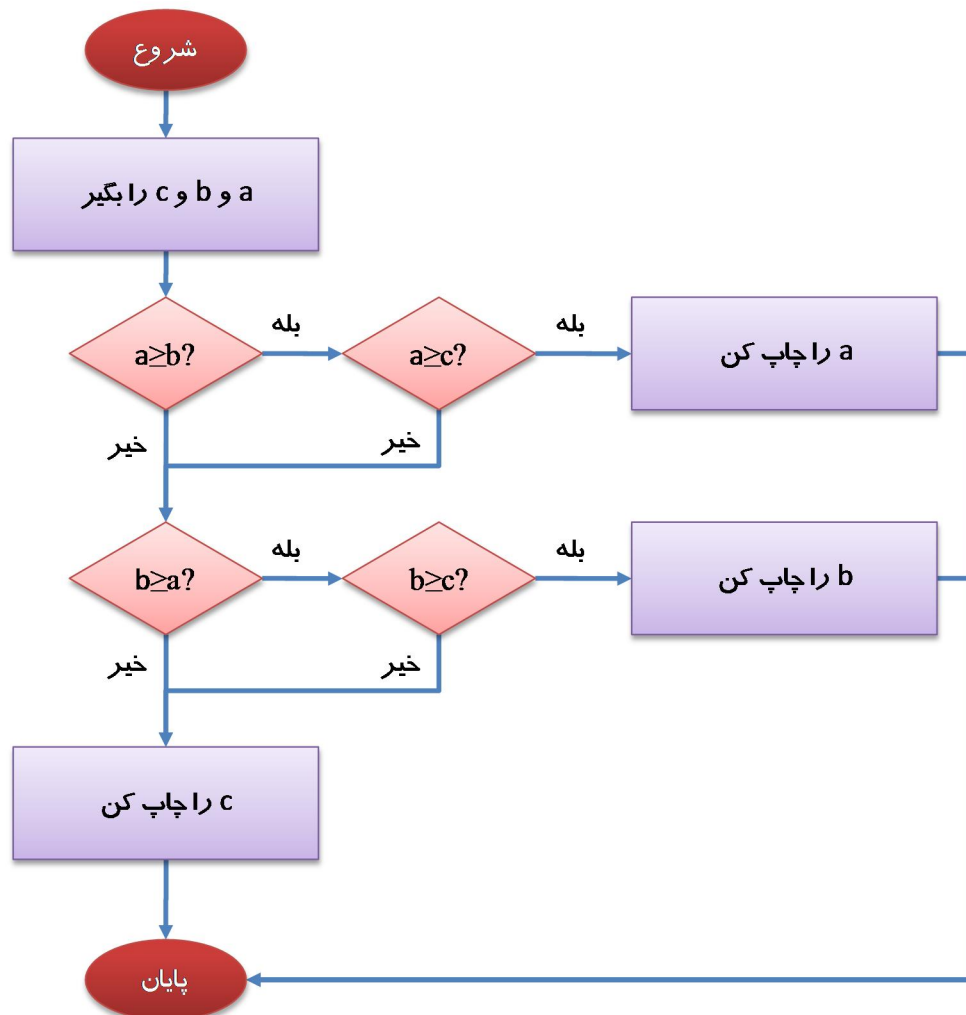
شکل ۲-۳: نمودار گردش حل مسأله‌ی یافتن بیشینه از بین سه عدد بدون استفاده از متغیر چهارم
