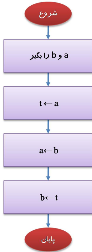
شکل ۷-۲: نمودار گردش تعویض محتوای دو متغیر با یکدیگر
