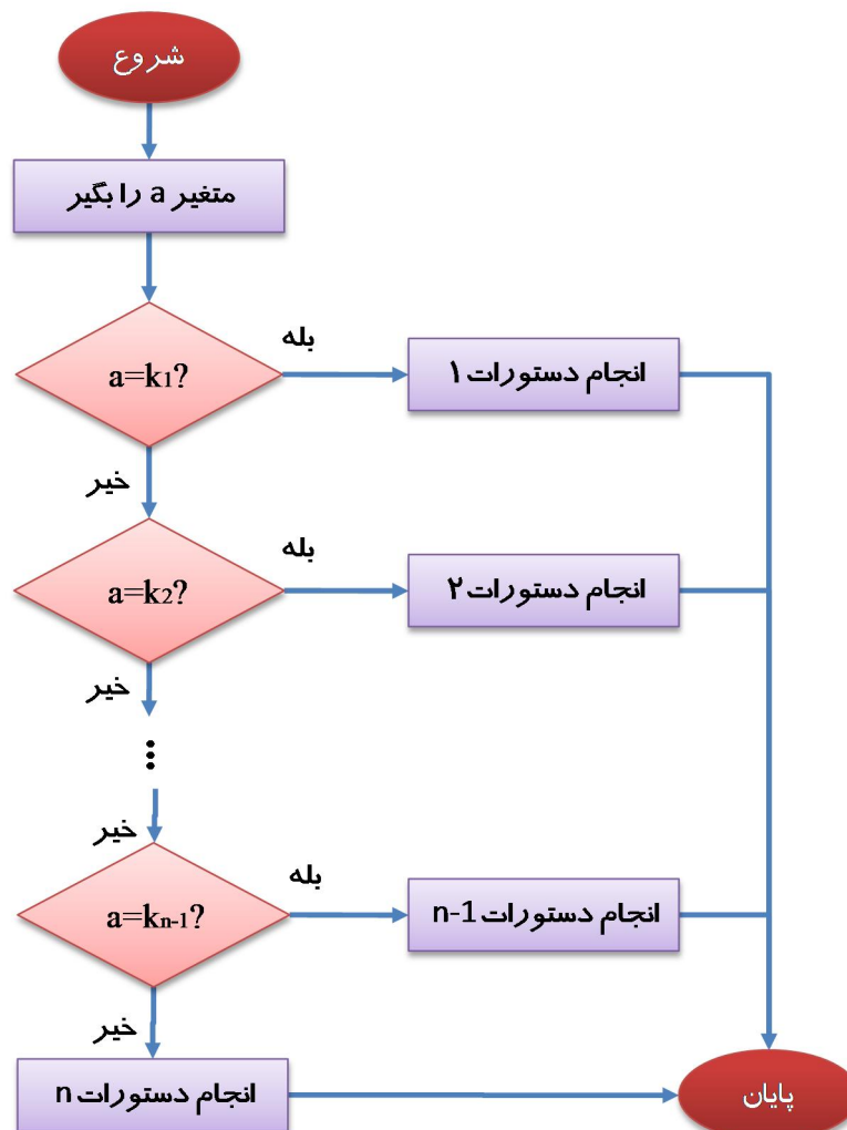
شکل ۳-۴: نمودار گردش‌ی ساختار تصمیم switch
