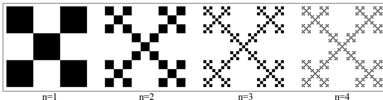
شکل ۱۰-۱۳: یک شکل خود متشابه به ازای n های مختلف. این شکل را می‌توان به صورت بازگشتی ترسیم کرد
