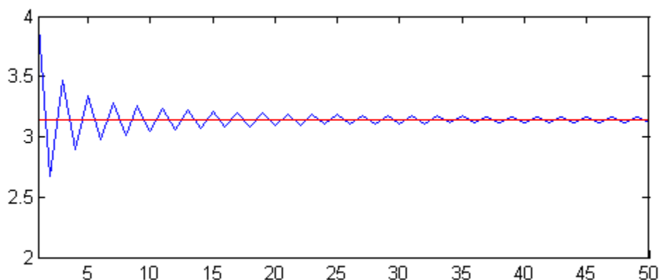
شکل ۶-۲: محاسبه‌ی عدد \pi تا ۵۰ جمله از روی رابطه‌ی تخمینی گفته شده (به کاهش خطای عدد به دست آمده بر حسب تعداد جملات دقت کنید).
