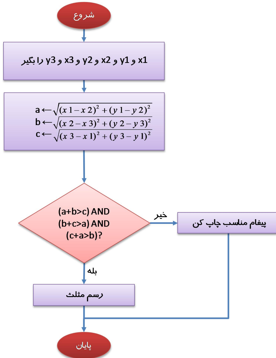
شکل ۵-۳: نمودار گردش‌ی گرفتن مختصات سه نقطه و ترسیم مثلث یا چاپ پیغام مناسب در صورت عدم تشکیل مثلث
