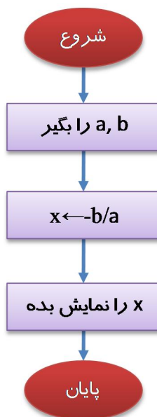
شکل ۳-۳: نمودار گردش حل معادله‌ی درجه اول بدون چک کردن شرط a \neq 0
