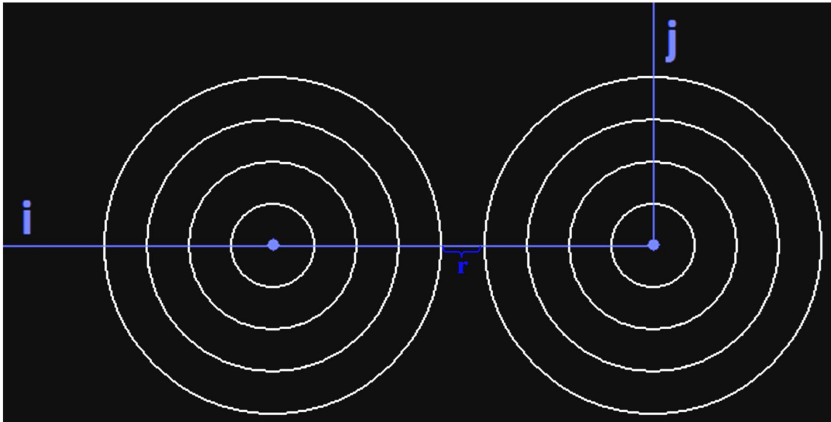
شکل ۵-۶: بررسی نحوه‌ی به دست آوردن مرکز دوائر متحدالمرکز واقع در سطر i و ستون j
