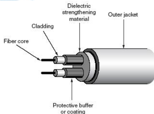
شکل ۳-۱۲ ساختمان فیبر نوری
