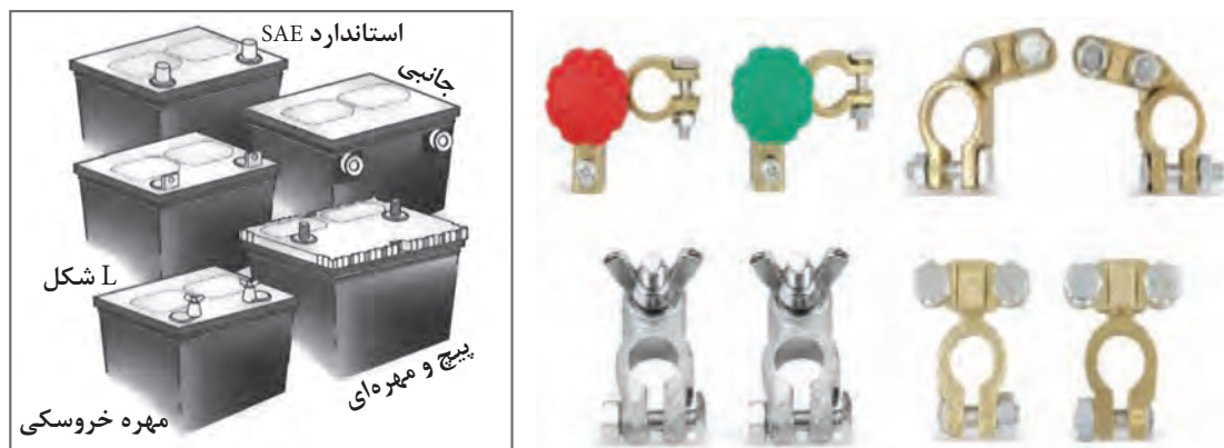
شکل ۳۱- چند نمونه بست باتری و روش اتصال آن به قطب‌ها
