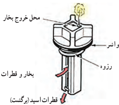
درپوش خانه باتری از نوع استاندارد
