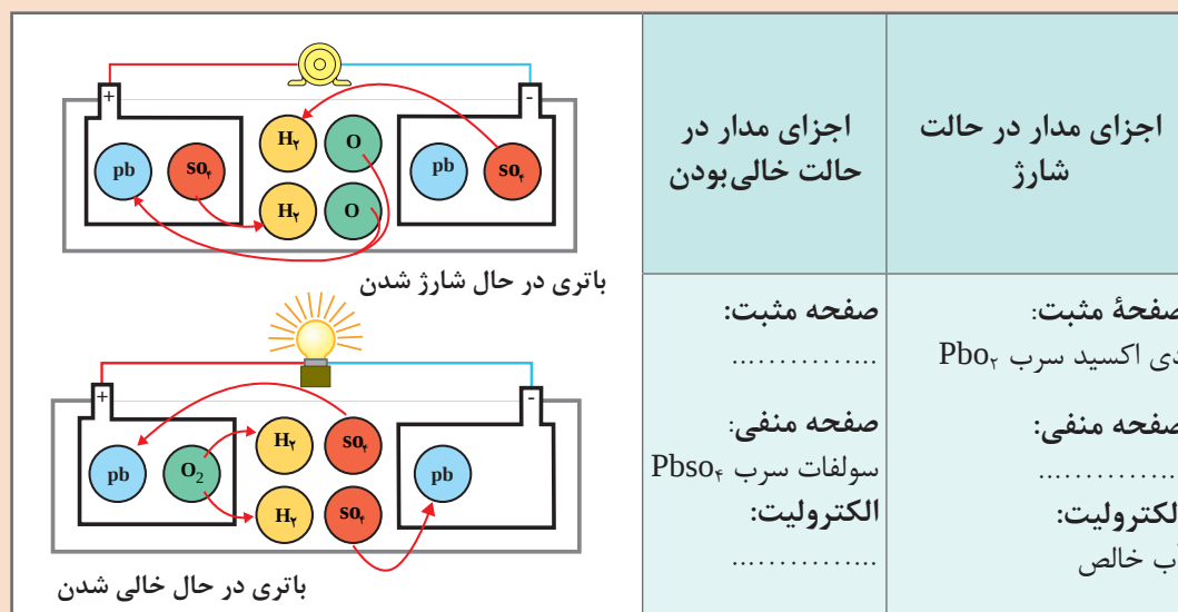
شکل ۱۷- واکنش‌های زمان شارژ و تخلیه باتری سربی اسیدی
