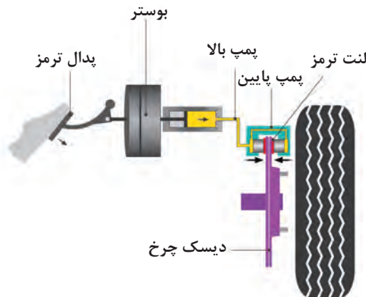
شکل ۳- شماتیک مکانیزم کارانداز سیستم ترمز
