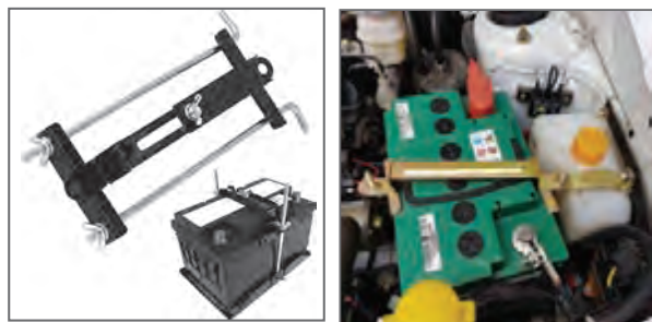
شکل ۳۲- چند نمونه از نگهدارنده‌های باتری
