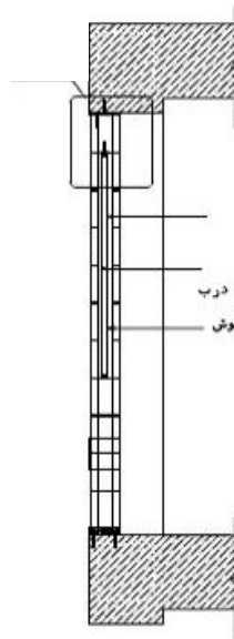
برش A-A
