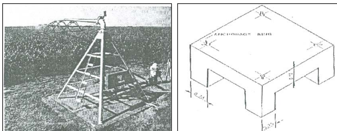
شکل ۸-۱۰- فونداسیون نقطه مرکزی دستگاه آب‌فشان دوار
