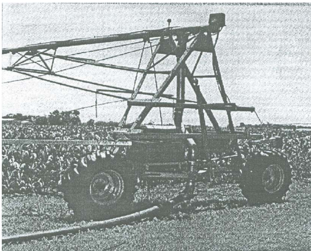
شکل ۸- ۱۱- آب‌گیری از طریق لوله تحت‌فشار زیرزمینی و شیلنگ
