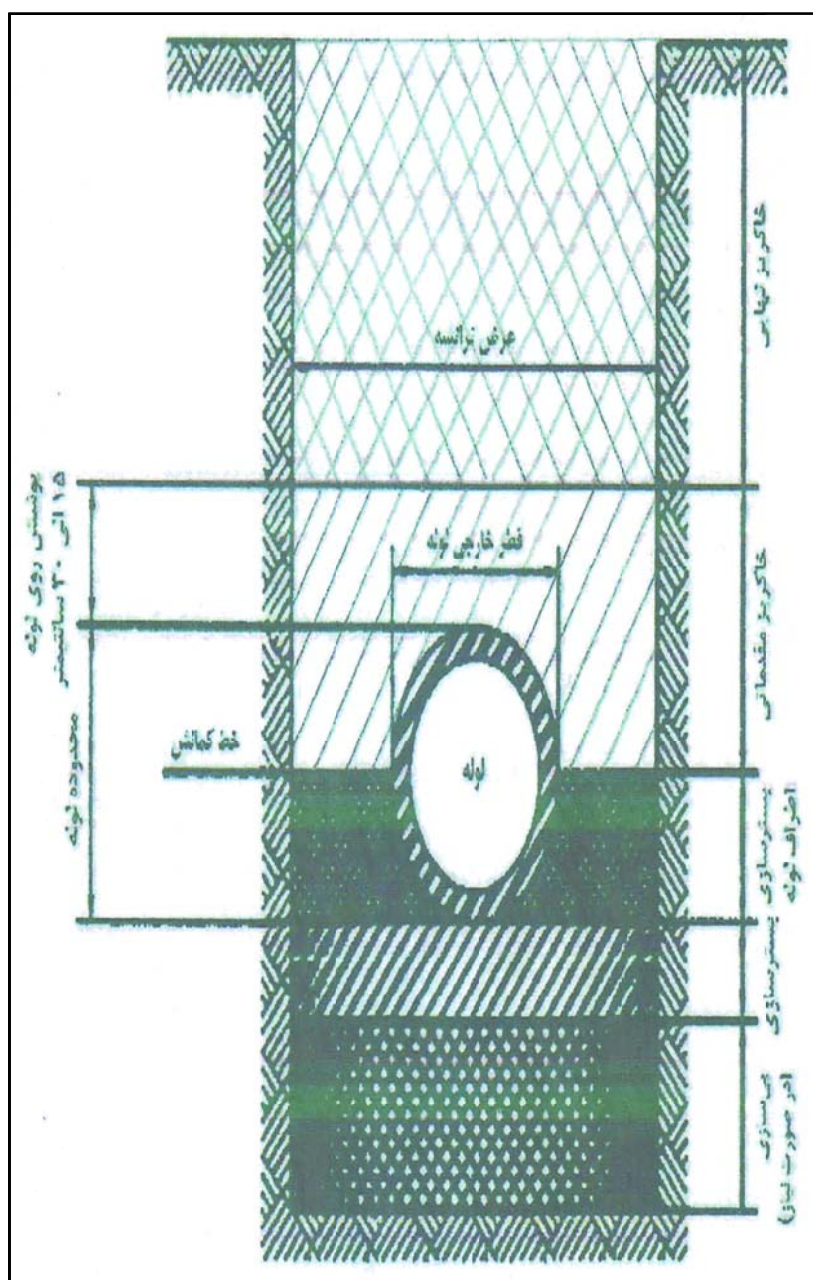
شکل ۶-۳- مقطع عرضی کارگذاری لوله پلی اتیلن
