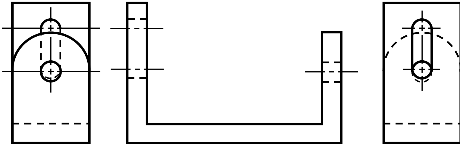
نمای اصلی
