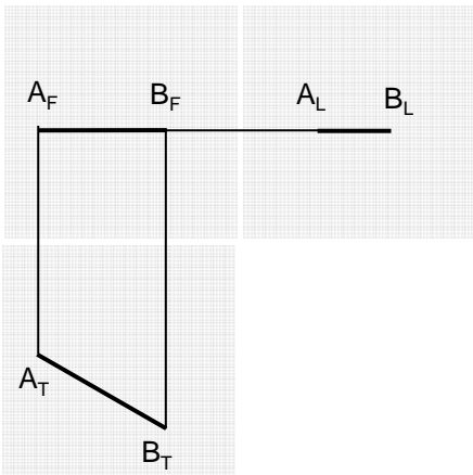
خط موازی
