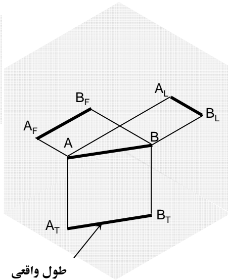
خط موازی
