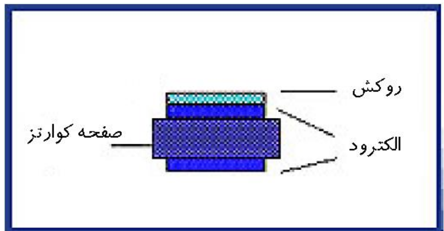
ساختمان یک QCM (Quartz Crystal Microbalance)
