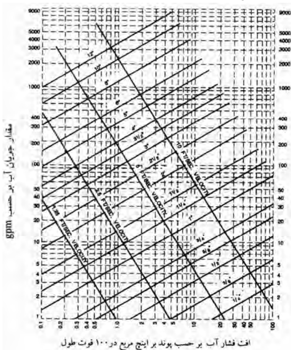
شکل پ ۱-۵-۵ (IP) منحنی اندازه‌گذاری لوله‌های مسی نوع K از استاندارد ANSI B ۸۸
