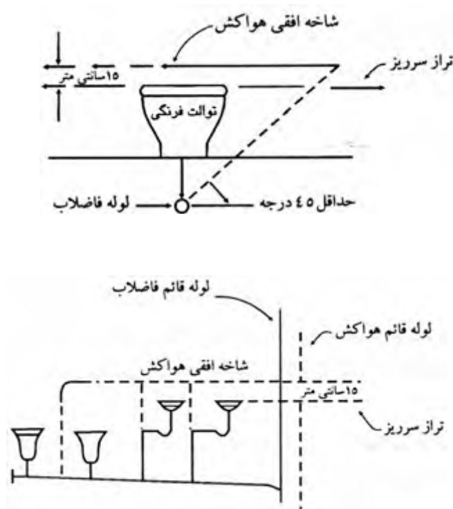
(شکل ۱۶ - ۶ - ۲ - ۵ - پ) (۲) اتصال هواکش به شاخه افقی لوله فاضلاب
