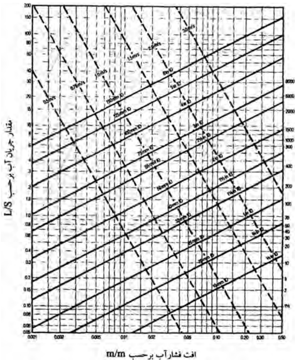
شکل پ - ۱ - ۵ - ۴ ت ۴ (SI) منحنی اندازه‌گذاری لوله‌های فولادی گالوانیزه
