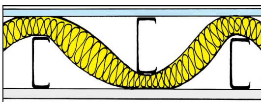
شکل ۴-۱۱- مقطع دیوار LSF با عایق حرارتی سینوسی
