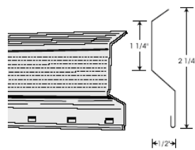
شکل ۱-۵- پروفیل ارتجاعی
