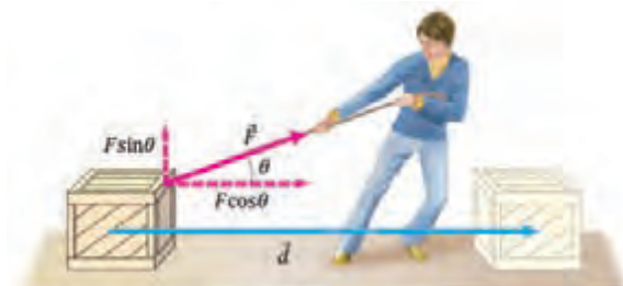
شکل ۳-۳ نیروی ثابت \vec{F} با جابه‌جایی \vec{d} زاویه \theta می‌سازد و کار W = (F \cos \theta) d را روی جسم انجام می‌دهد.
