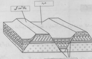
چین‌خوردگی رسوبات
