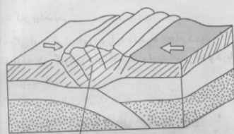
شکستگی (گسل)
