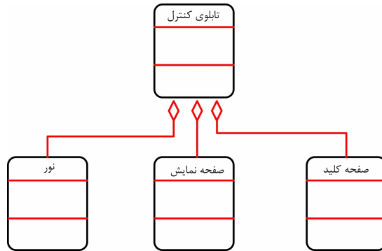
شکل ۱۱-۷ نمودار کلاس‌ها برای کلاس‌های مجتمع مرکب
