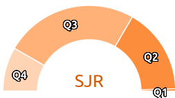
توزیع مقالات در چارکها براساس شاخص SJR
