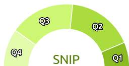
توزیع مقالات در چارکها براساس شاخص SNIP
