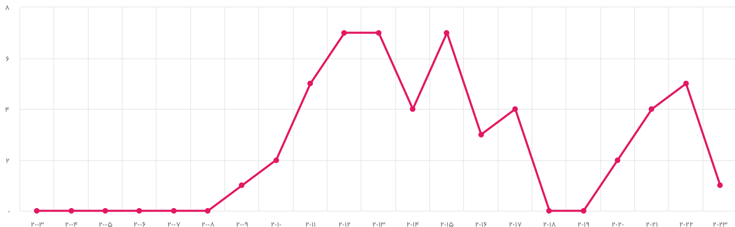
تعداد مقالات (منتشر شده در سال مشخص)
