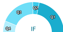
توزیع مقالات در چارکها براساس شاخص IF
