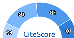
توزیع مقالات در چارکها براساس شاخص CiteScore
