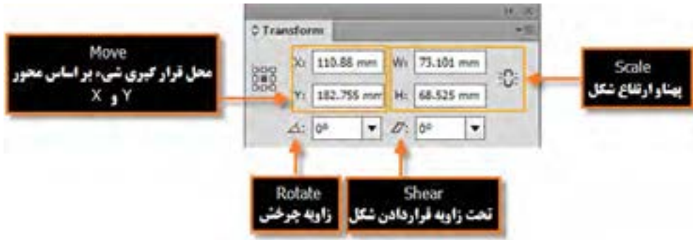
شکل ۴-۳۳ پنل Transform
