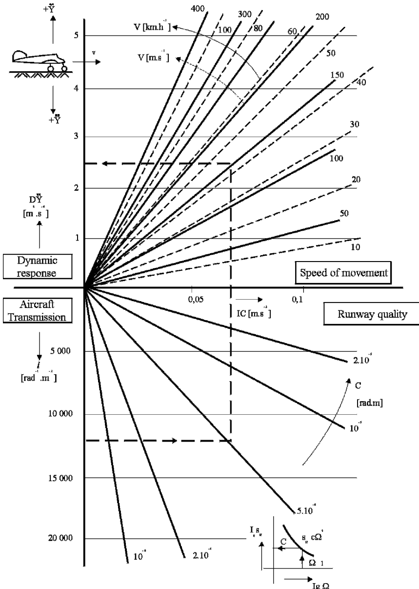
Figure 8-15 Dynamic response of aircraft vertical acceleration on different pavement quality (Source: Čihař, J.: Letiště a jejich zařízení, Alfa Bratislava 1973)
