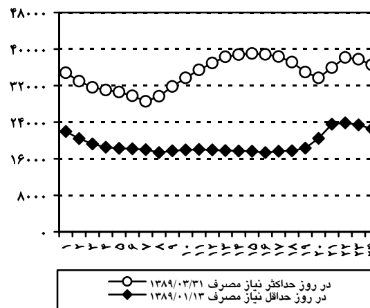
نمودار (۴-۴): تغییرات ۲۴ ساعته نیاز مصرف اصلاح شده
