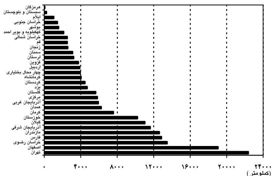
نمودار (۱-۳): طول شبکه گذاری گاز طبیعی استان‌های کشور تا پایان سال ۱۳۸۹
