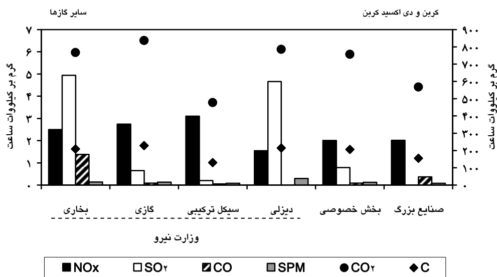
نمودار (۸-۳): شاخص انتشار گازهای آلاینده و گلخانه‌ای از بخش نیروگاهی کشور در سال ۱۳۸۹
