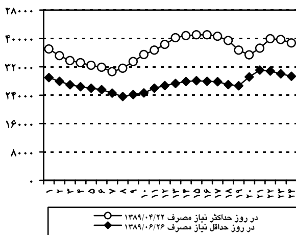
نمودار (۴-۵): تغییرات ۲۴ ساعته نیاز مصرف اصلاح شده شبکه
