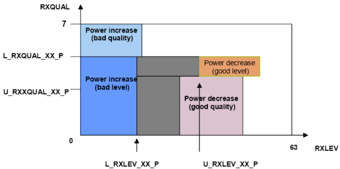
شکل (3-16): سطوح تریگر کنترل توان افقی
