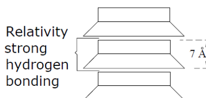
شکل ۱-۸ نحوه پیوند واحدهای پایه کانی کائولینیت
