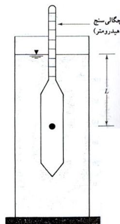
شکل ۱-۱۷ تعریف طول موثر L در آزمایش هیدرومتری
