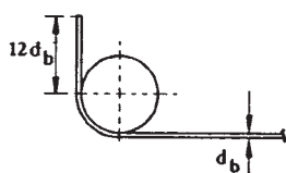
خم انتهایی ۹۰ درجه (گونیا)
