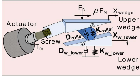
Fig. 3. EWB model.
