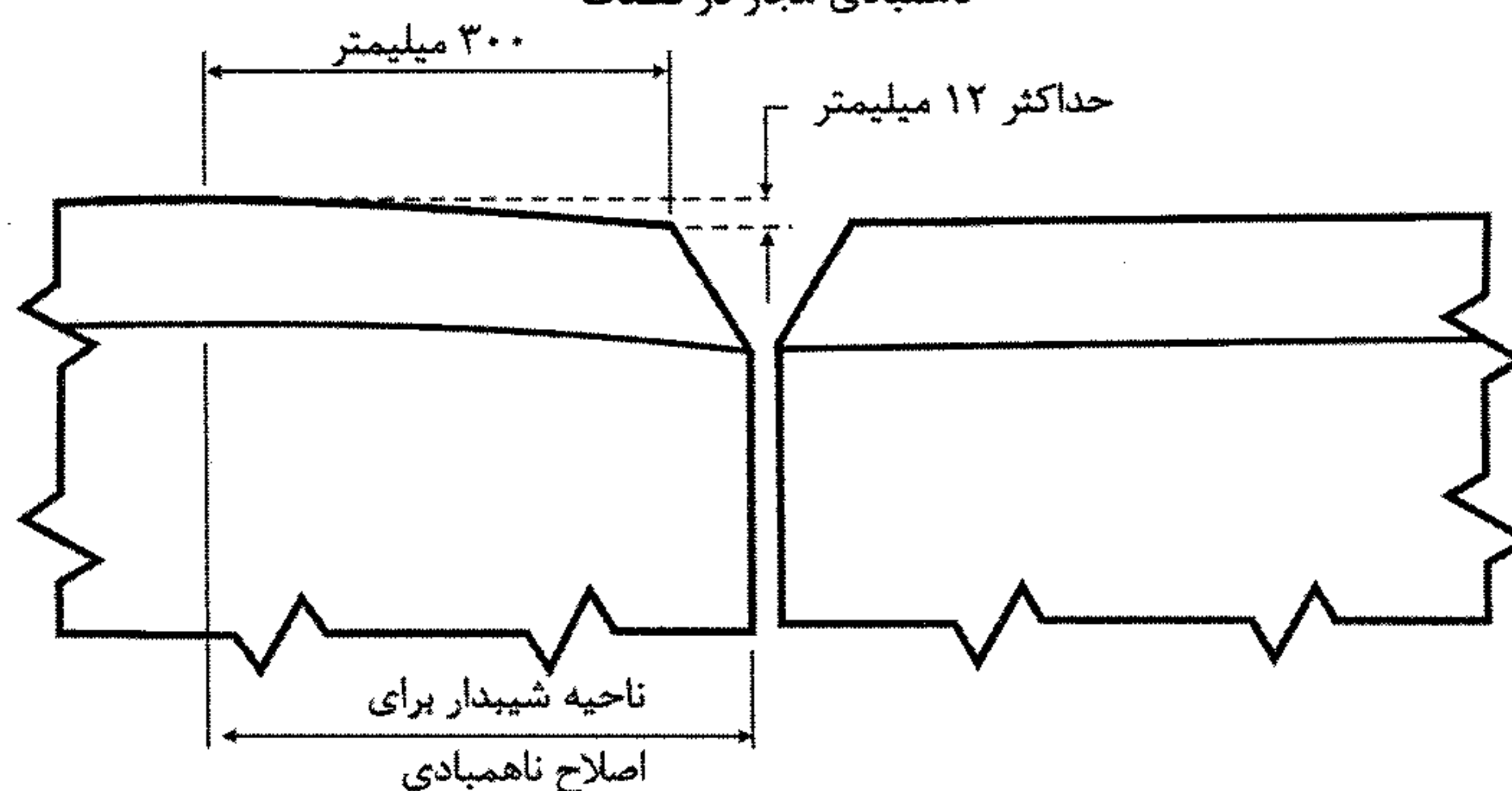
شکل ۶-۴-۱۰ اصلاح ناهمبادی و ناهم‌محوری
