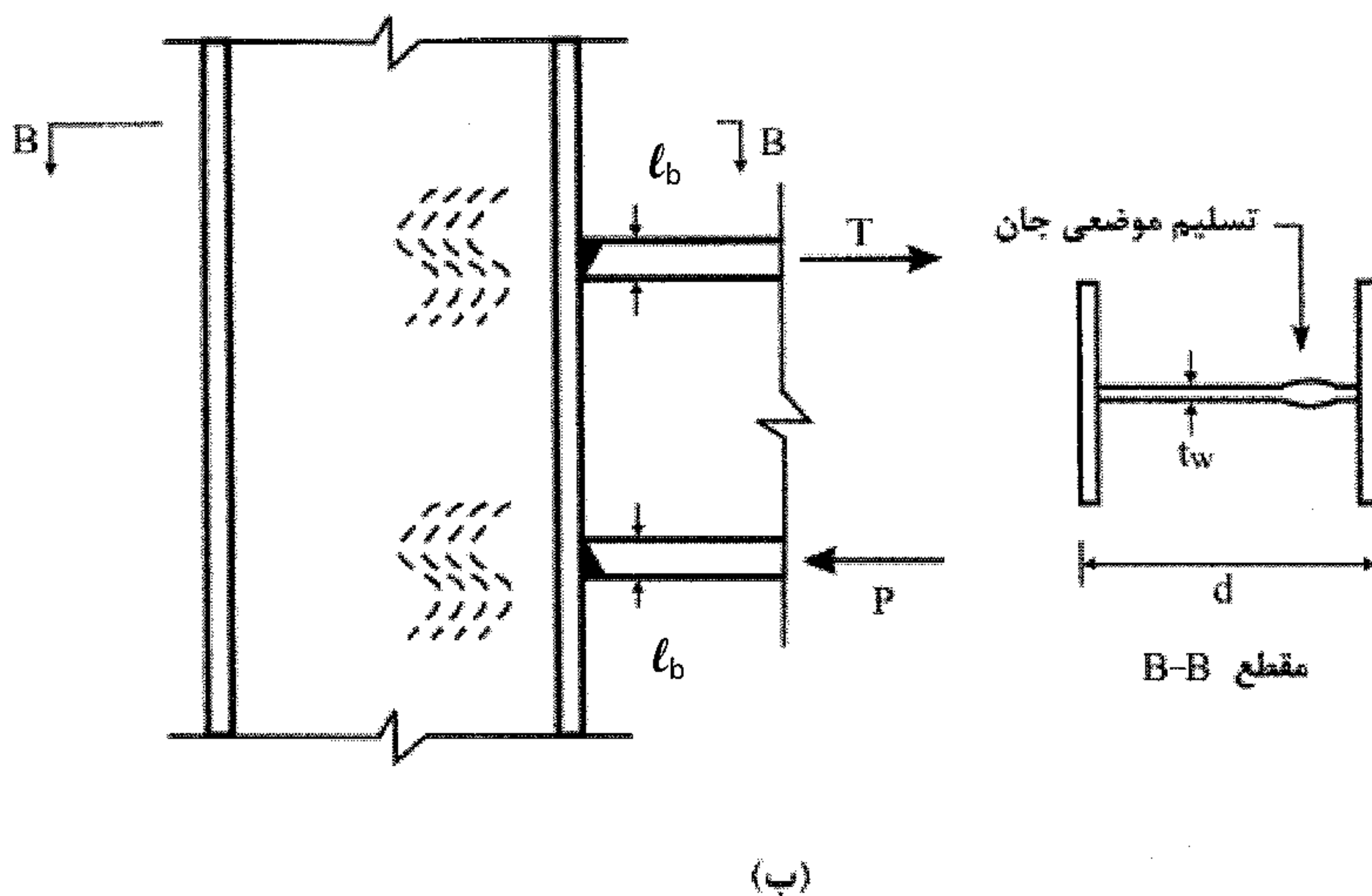
شکل ۱۰-۲-۹-۱۷ تسلیم موضعی جان در مقابل نیروی متمرکز کششی و فشاری
