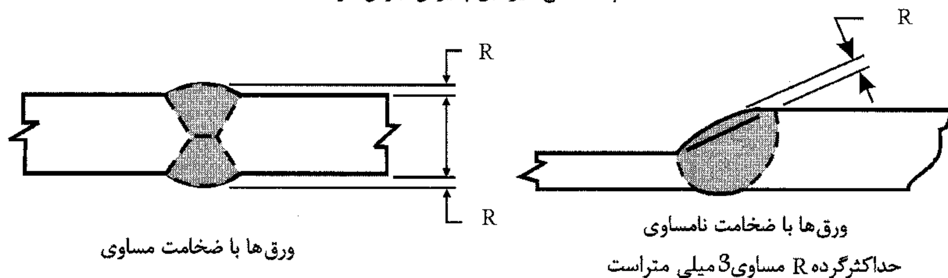
(ت) مقاطع قابل پذیرش جوش های شیاری
