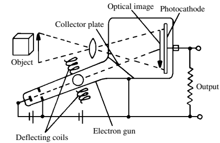
iconoscope
