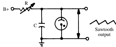
gas-tube oscillator
