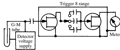
Geiger counter
