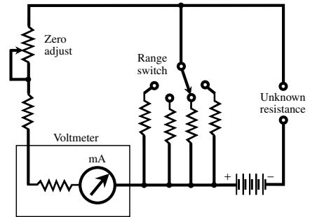
ohmmeter
