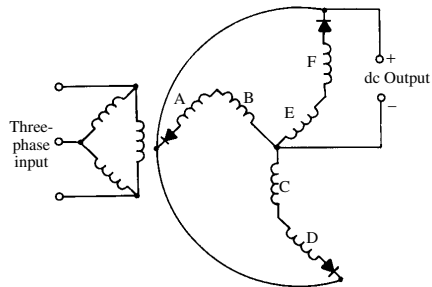
zigzag rectifier
