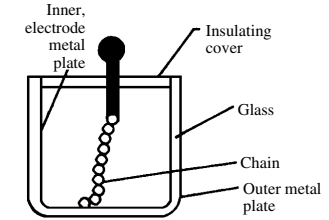
Leyden jar
