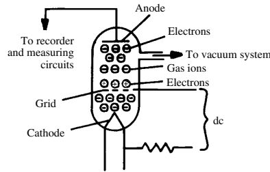
ionization gauge
