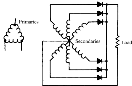
six-phase rectifier
