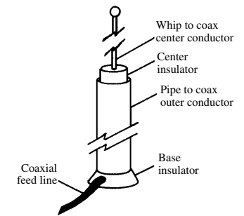
flagpole antenna, 1
