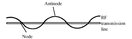
antinode
