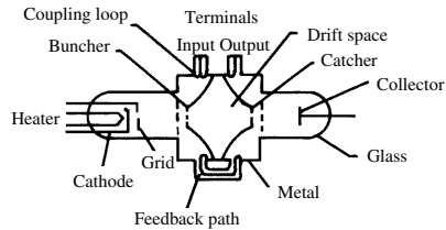
klystron
