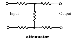
attenuator
