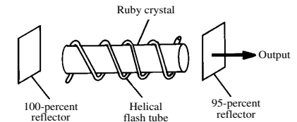
ruby laser
