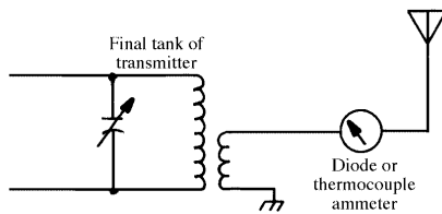
antenna ammeter
