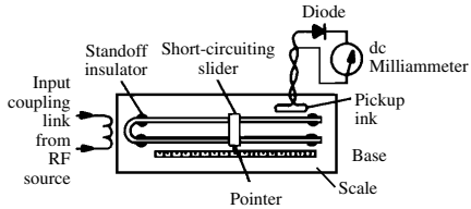
Lecher frame
