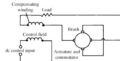
amplidyne
