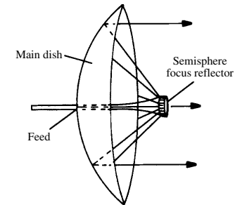
Cassegrain antenna
