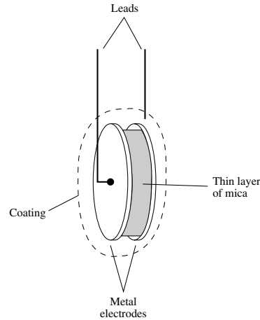
mica capacitor
