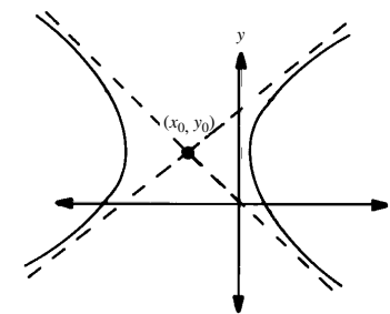
hyperbola
