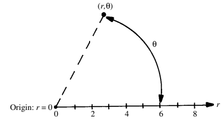
polar coordinates
