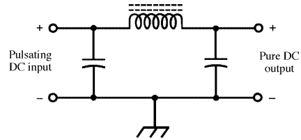
rectifier filter
