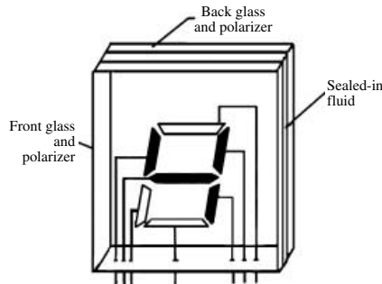
liquid-crystal display
