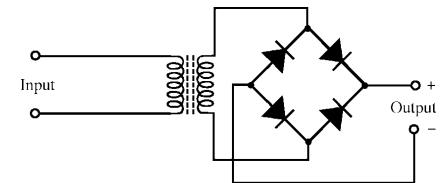
bridge rectifier
