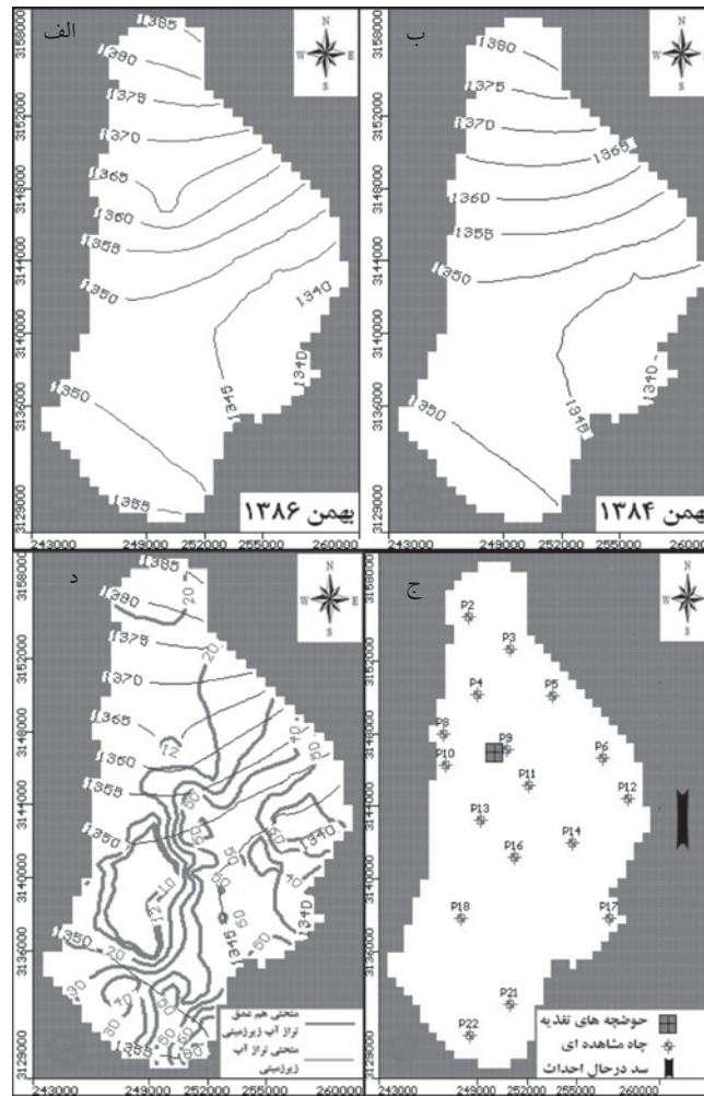
شکل ۱۴- الف) منحنی‌های تراز بهمن ۸۴ ب) منحنی‌های تراز بهمن ۸۶ در حالت تغذیه مصنوعی ج) محل حوضچه‌های تغذیه، سد در حال ساخت و چاه‌های مشاهده‌ای (د) نقشه هم‌تراف و تراز آبی بهمن ۸۶ در حالت تغذیه مصنوعی به آبخوان با فرض تأمین آب تغذیه از سد
