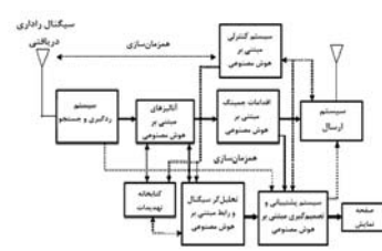
شکل شماره (۳) بلوک دیگرام سامانه EW تلفیق شده با AI
