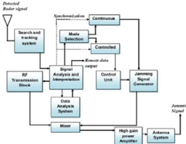
شکل شماره (۲) بلوک دیگرام سامانه EW نمونه
